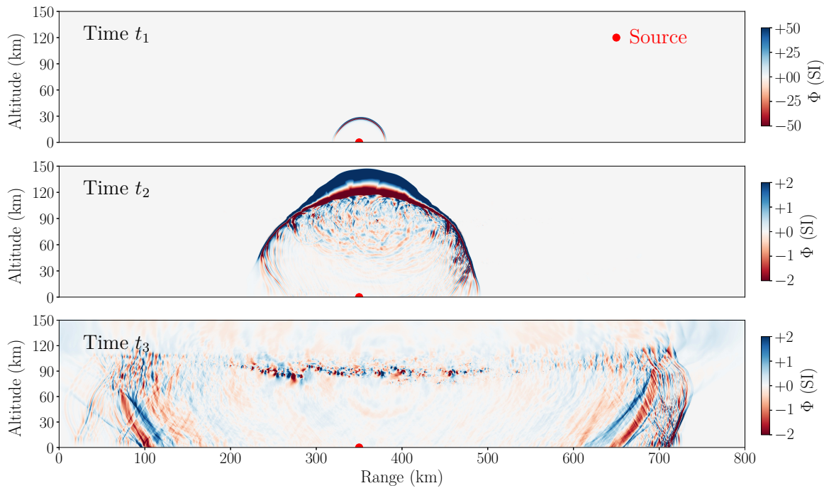
Figure 2: Perturbations de pression à différents instants de temps dues à une onde infrasonore émise au sol par une source impulsive et se propageant dans le champ turbulent induit par le déferlement d’une onde de gravité.
