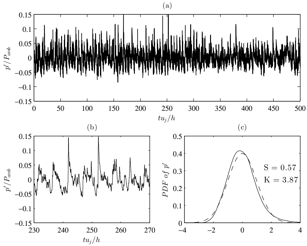
FIGURE 4.13 – Evolution temporelle de la pression fluctuante en x = 0 et y = 8.5h pour JetpL5 : (a) sur toute la durée de la simulation et (b) sur une période de 40h/u_j s; (c) densité de probabilité — de la pression fluctuante et — — — d'une distribution gaussienne.
