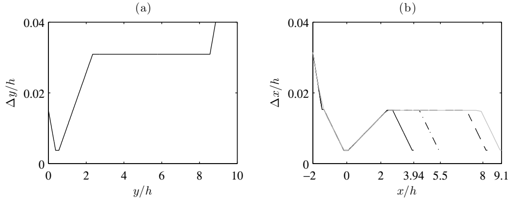
FIGURE 4.3 – Evolution de la taille des mailles dans les directions (a) latérale et (b) axiale pour — JetpL3, —·— JetpL5, — — — JetpL8, et — JetpL9.
