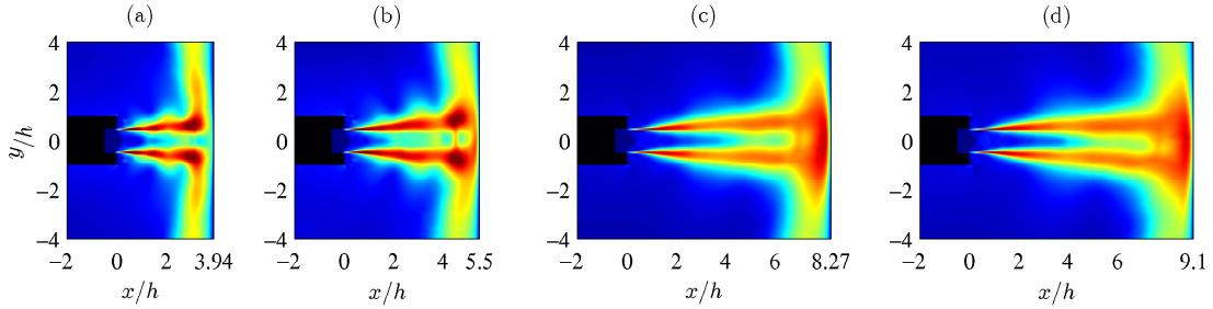
FIGURE 4.8 – Champs rms de la vitesse axiale dans le plan (x, y) pour (a) JetpL3, (b) JetpL5, (c) JetpL8 et (d) JetpL9. L'échelle de couleur varie pour des valeurs de 0 à 100 m.s -1 . La buse est en noir.
