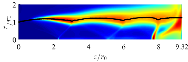
FIGURE 3.33 – Vitesse rms totale pour JetL9. L'échelle de couleur varie pour des valeurs de 0 à 100m.s -1 . La ligne noire indique le chemin suivant lequel a été calculé la vitesse de convection.
