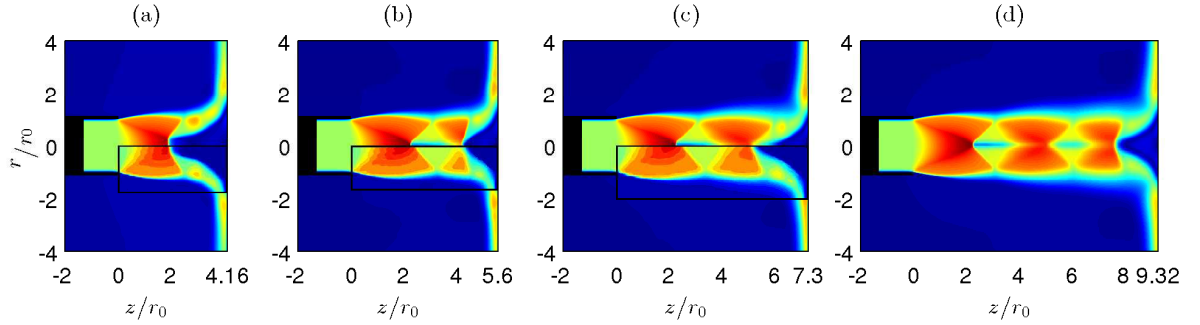
FIGURE 3.27 – Champs moyens de vitesse totale dans le plan (z, r) pour (a) JetL4, (b) JetL5, (c) JetL7 et (d) JetL9. L'échelle de couleur varie pour des valeurs de 0 à 500\text{m.s}^{-1} . Les résultats expérimentaux de Henderson et al. [59] sont représentés dans les rectangles noirs.
