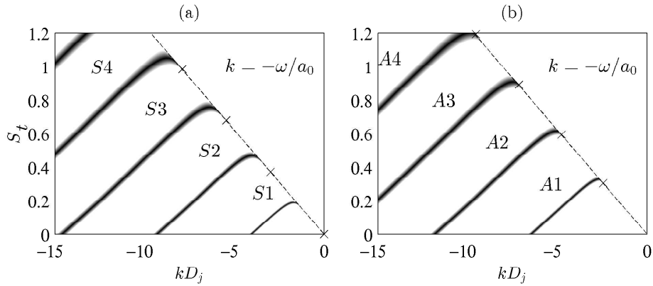
FIGURE 1.17 – Relation de dispersion des modes acoustiques neutres (a) axisymétrique et (b) hélicoïdaux du jet rond idéalement détendu équivalent à un jet issue d'une tuyère convergente avec \mathcal{M}_j = 1.56 et r_0 = 1\text{mm} ; \times limites basses des modes et - - - k = -\omega/a_0 .
