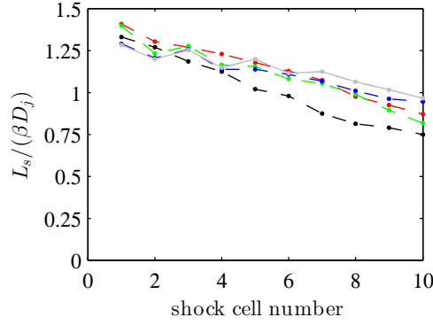
FIGURE 3.8 – Taille normalisée des dix premières cellules du réseau de cellules de chocs pour – ● – le jet libre simulé et les jets expérimentaux de André et al. [3] à des nombres de Mach parfaitement détendus de – ● – \mathcal{M}_j = 1.10 , – ● – \mathcal{M}_j = 1.15 , – ● – \mathcal{M}_j = 1.35 et – ● – \mathcal{M}_j = 1.50 .
