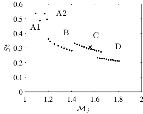
FIGURE 3.18 – • Représentation des fréquences dominantes du bruit de screech obtenues expérimentalement par Powell et al. [113] en fonction du nombre de Mach du jet équivalent idéalement adapté \mathcal{M}_j ; × fréquence dominante du screech obtenue pour le jet simulé.
