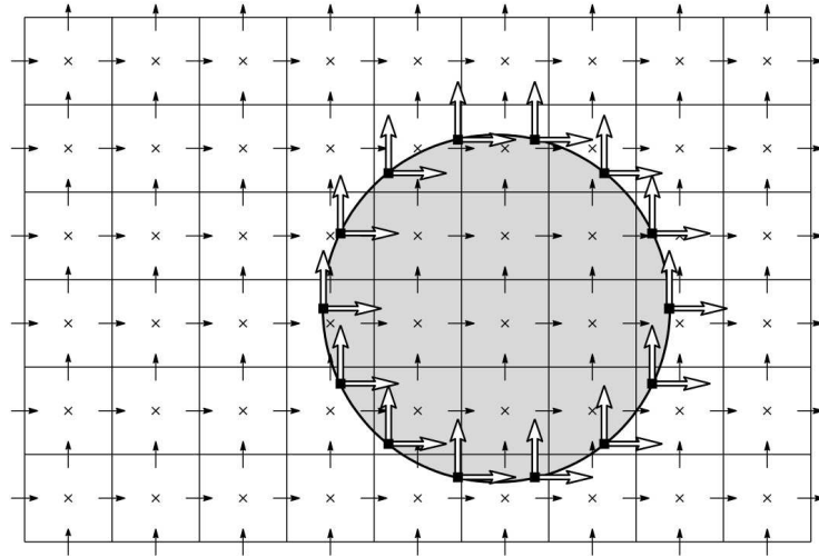
FIGURE 2.7 – Méthode discrète proposée par Taira et Colonius [133] sur un maillage structuré. Le fluide est représenté en blanc et le solide est représenté en gris; \times et \rightarrow composantes de la pression et de la vitesse venant de la discrétisation des équations de Navier-Stokes sur le maillage; \blacksquare points de la paroi et \Rightarrow termes sources reproduisant les effets de la paroi.
