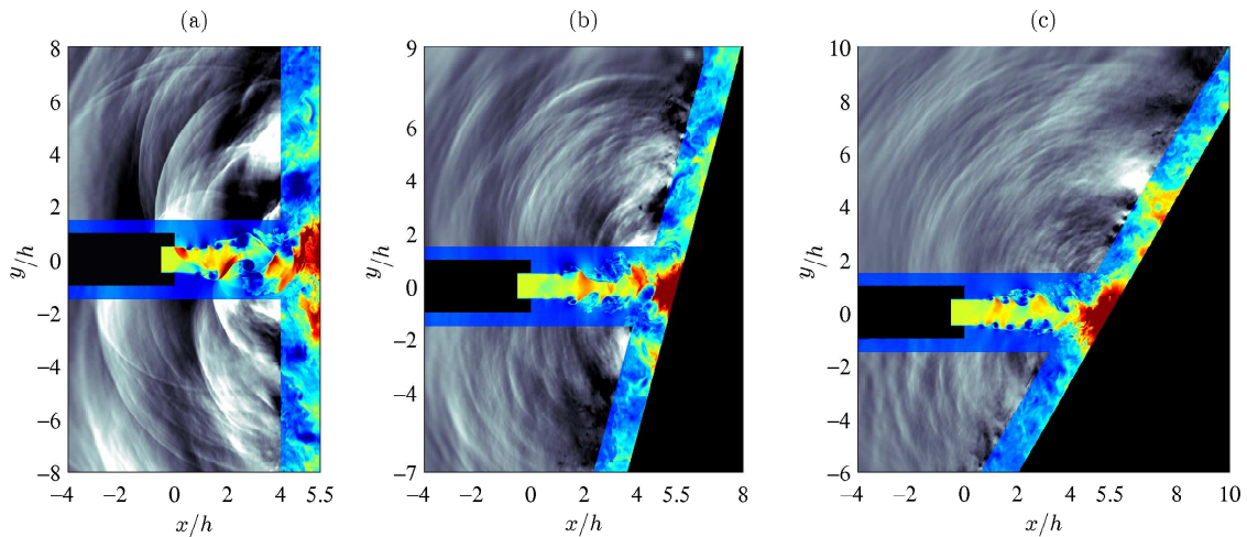
FIGURE 4.27 – Représentations instantanées dans le plan (x, y) de la masse volumique dans les régions proches du jet et de la paroi, et de la pression fluctuante pour (a) JetpL5, (b) JetpL5-75d et (c) JetpL5-60d. Les échelles de couleur varient pour des valeurs de 1 à 2 \text{ kg.m}^{-3} pour la masse volumique et de -7500 à 7500 \text{ Pa} pour la pression fluctuante. La buse et la paroi sont en noir.
