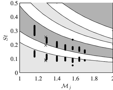
FIGURE 4.16 – Plages de fréquences envisageables pour les deux premiers modes symétriques en gris clair et antisymétriques en gris foncé; • données expérimentales de Tam et Norum [143], × fréquences tonales dominantes des quatre jets.
