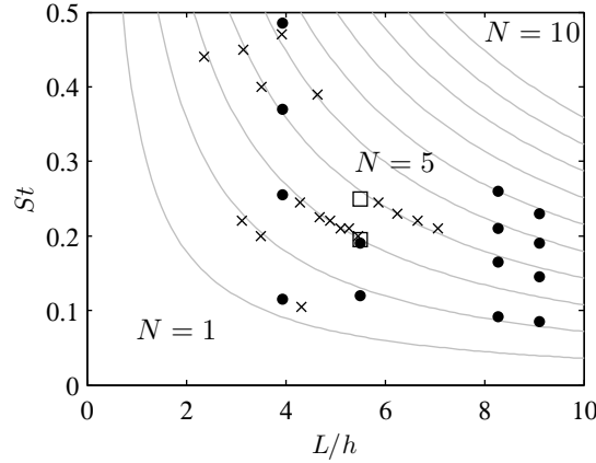
FIGURE 4.32 – Nombre de Strouhal des fréquences tonales obtenues pour • les jet JetpL3, JetpL5, JetpL8 et JetpL9, □ pour JetpL5-75d et × expérimentalement par Thurow et al. [153] pour des jets aux conditions d'éjections similaires. — représente les valeurs prédites par la relation (1.32) en considérant \langle u_c \rangle = 0.60u_j .
