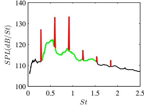
FIGURE 1.5 – Spectre acoustique d'un jet supersonique sous-détendu avec un nombre de Mach parfaitement détendu de \mathcal{M}_j = 1.35 et un nombre de Reynolds de 10^6 [2], obtenu à un angle de 110 degrés par rapport à la direction du jet : — screech, — bruit de choc large bande.
