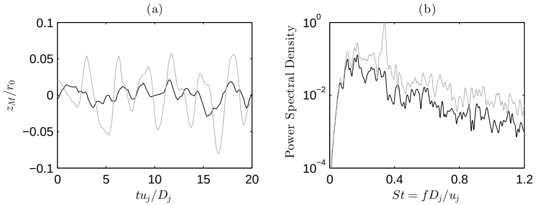
FIGURE 3.45 – (a) Position axiale du choc z_M au cours du temps et (b) densité spectrale de puissance de cette position pour jetL9; — résultats pour le disque de Mach sur l’axe du jet, et — résultats pour le disque de Mach sur la ligne r = 0.7r_0 . L’échelle de la densité spectrale de puissance est arbitraire.
