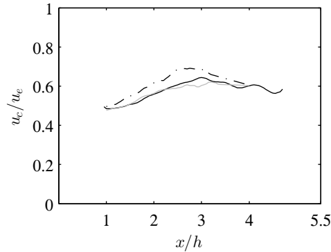
FIGURE 4.30 – Vitesse de convection des structures turbulentes le long de la couche de mélange en y = -h/2 pour — JetpL5, — JetpL5-75d et -.- JetpL5-60d.
