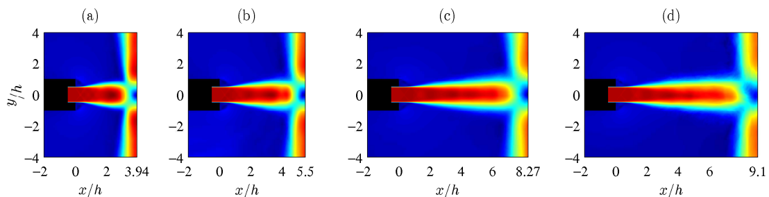
FIGURE 4.7 – Champs moyens de vitesse totale dans le plan (x, y) pour (a) JetpL3, (b) JetpL5, (c) JetpL8 et (d) JetpL9. L'échelle de couleur varie pour des valeurs de 0 à 400 m.s^{-1} . La buse est en noir.
