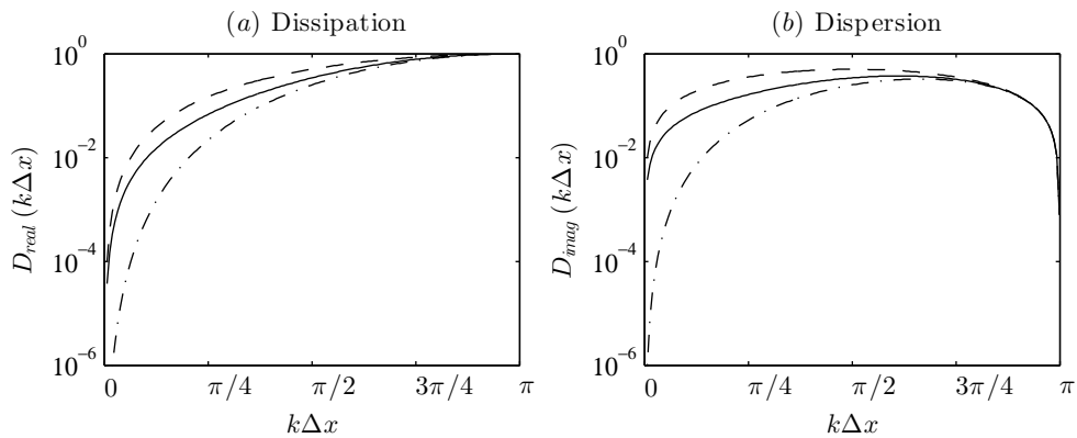
FIGURE 2.5 – Fonctions de transfert du filtrage non-linéaire en fonction du nombre d'onde k\Delta x . (a) Dissipation et (b) dispersion pour — le filtre optimisé d'ordre 2, -.- le filtre standard d'ordre 4 et - - - le filtre standard d'ordre 2.
