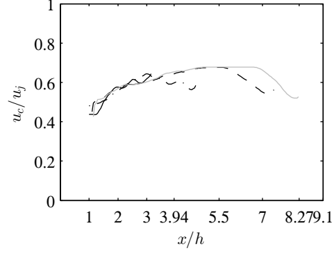
FIGURE 4.11 – Vitesse de convection des structures turbulentes le long des couches de mélange des jets pour — JetpL3, -·- JetpL5, - - - JetpL8, et — JetpL9.
