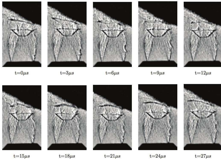
FIGURE 1.22 – Images shadowgraph montrant le cycle complet d'un mode de flexion/battement pour un jet rond impactant une paroi située en 2D avec un angle de 60 degrés et avec un taux de détente de 4.5, d'après Risborg et Soria [116].
