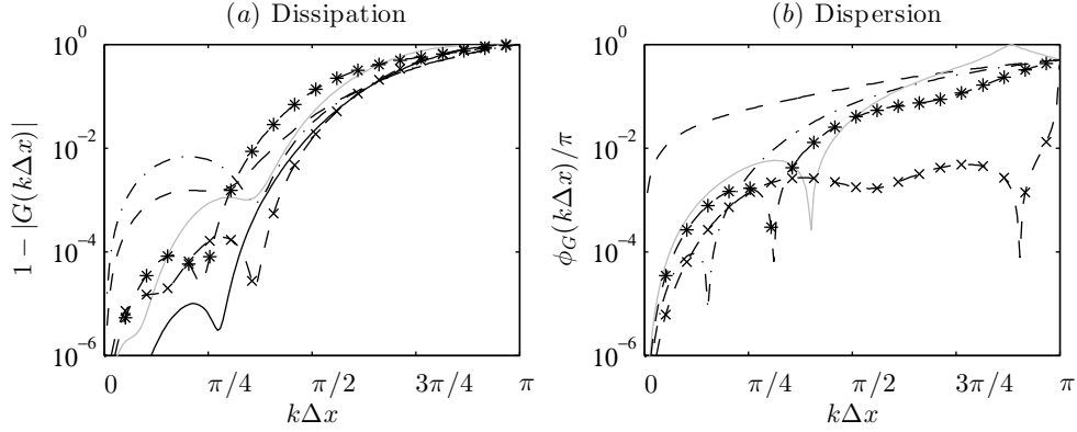
FIGURE 2.3 – Filtres centrés de Bogey et al. [22] et décentrés de Berland et al. [12]. (a) Dissipation et erreur de (b) dispersion en fonction du nombre d'onde k\Delta x . — Filtre centré SFo11p, — — — filtre décentré SFo010d, — · — filtre décentré SFo19d, — — — filtre décentré SFo28d, — * — filtre décentré SFo37d et — × — filtre décentré SFo46d.
