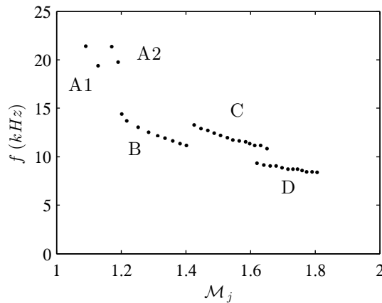
FIGURE 1.6 – Evolution de la fréquence fondamentale du bruit de screech en fonction du nombre de Mach parfaitement détendu \mathcal{M}_j , • données expérimentales de Powell et al. [113].
