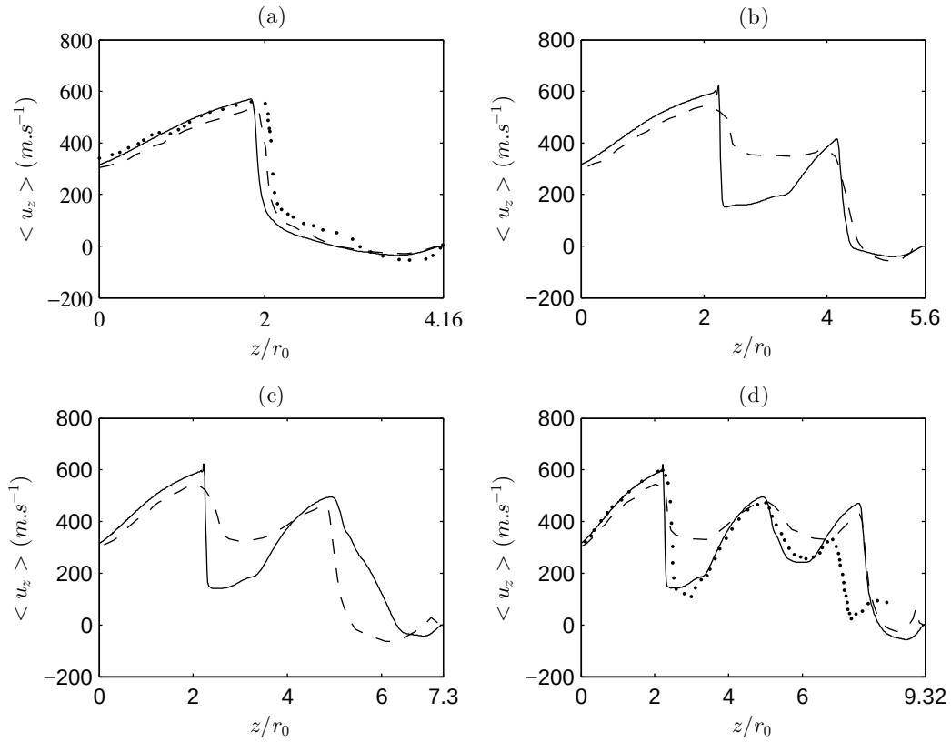
FIGURE 3.28 – Vitesses moyennes axiales sur l’axe des jets en fonction de la direction axiale pour (a) JetL4, (b) JetL5, (c) JetL7 et (d) JetL9; — résultats des simulations, — — — résultats expérimentaux de Henderson et al. [59], et • résultats numériques de Dauplain et al. [37, 38] pour des distances entre la buse et la paroi égales à (a) 4.16r_0 et (d) 8.32r_0 .
