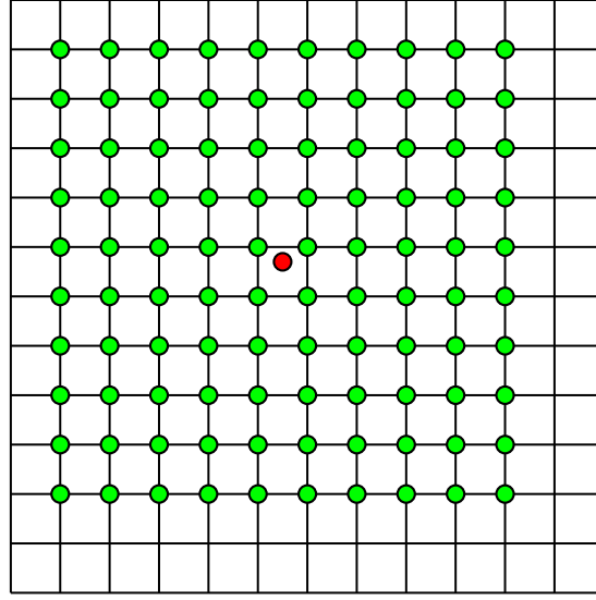
FIGURE 2.10 – Méthode d'interpolation à l'aide de polynômes de Lagrange en 2-D; ● point receveur et ● points donneurs.
