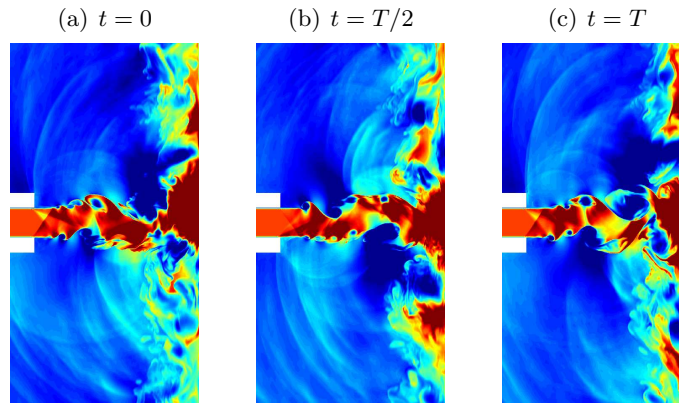
FIGURE 1.15 – Représentation instantanée de la masse volumique obtenue par un jet supersonique rectangulaire adapté impactant une paroi avec un angle normal, pour un nombre de Mach d'éjection de 1.28 et un nombre de Reynolds de 5.10^4 ; simulation des grandes échelles présentée dans le chapitre 4; T est la période fondamentale du mode sinueux.
