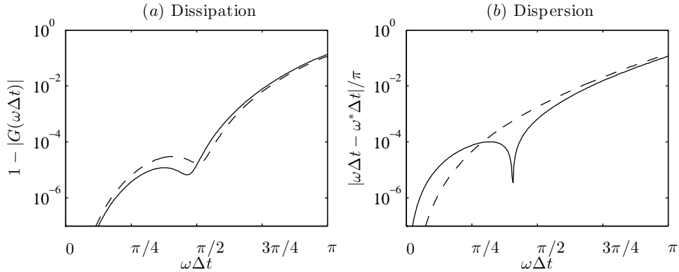
FIGURE 2.2 – Algorithme de Runge-Kutta. Erreurs de (a) dissipation et (b) dispersion en fonction de la pulsation \omega\Delta t : — RK26 de Bogey et Bailly [16] et - - - RK46 de Berland et al. [10].
