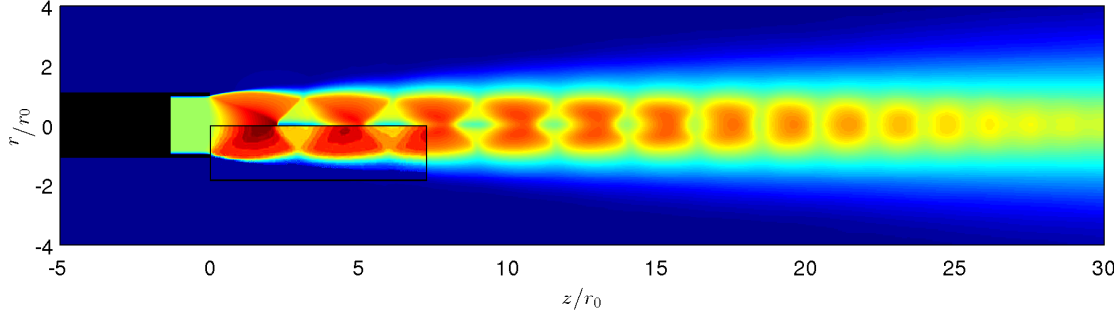
FIGURE 3.7 – Champs moyens dans le plan (z, r) de la vitesse totale. L'échelle de couleur varie pour des valeurs de 0 à 600 m.s -1 . Les résultats PIV de Henderson et al. [59] pour un jet supersonique sous-détendu ( \mathcal{M}_j = 1.56 et \mathcal{M}_e = 1 ) sont montrés dans le rectangle noir.
