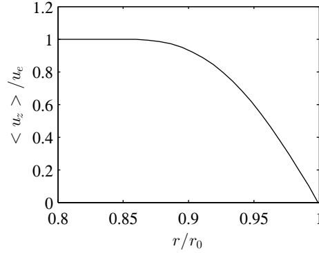
FIGURE 3.1 – Profil de vitesse moyenne axiale en sortie de la buse.
