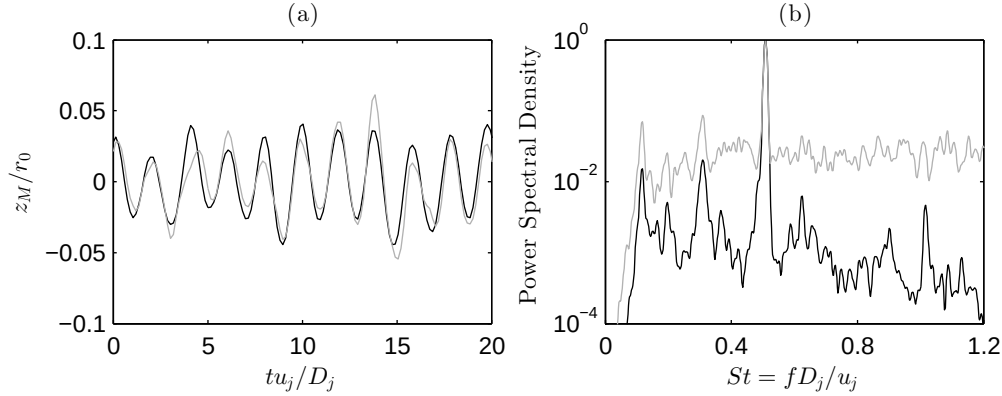
FIGURE 3.43 – (a) Position axiale du choc z_M au cours du temps et (b) densité spectrale de puissance de cette position pour jetL4; — résultats pour le disque de Mach sur l’axe du jet, et - - - résultats pour le choc oblique sur la ligne r = 0.7r_0 . L’échelle de la densité spectrale de puissance est arbitraire.
