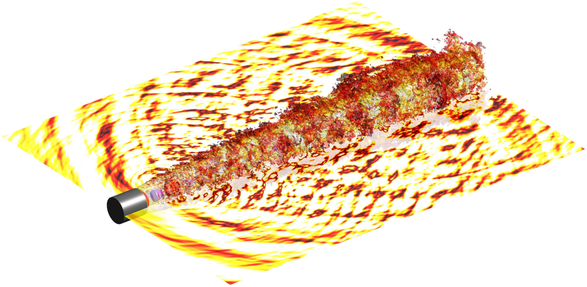
FIGURE 3.3 – Visualisation du jet simulé. Les isosurfaces de masse volumique en mauve et rouge sont obtenues pour des valeurs 0.8 et 2.5 \text{ kg.m}^{-3} , respectivement. Les isosurfaces de masse volumique correspondant à 1.25 \text{ kg.m}^{-3} sont également représentées et sont colorées par le nombre de Mach local. Le champ de pression fluctuante dans le plan \theta = 0 degré est montré. La buse est en gris.
