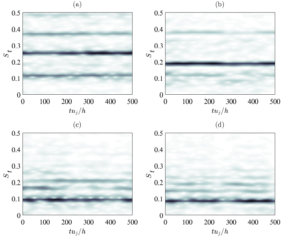
FIGURE 4.25 – Spectres acoustiques au point de coordonnées x = 0 et y = 1.5h en fonction du temps et du nombre de Strouhal pour (a) JetpL3, (b) JetpL5, (c) JetpL8 et (d) JetpL9.
