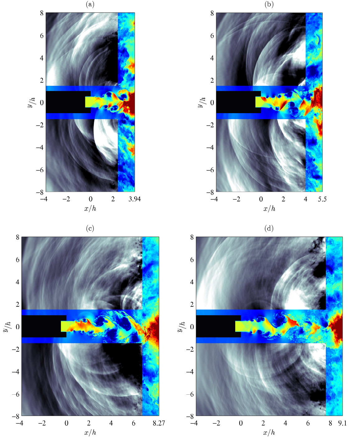
FIGURE 4.6 – Représentations instantanées dans le plan (x, y) de la masse volumique dans les régions proches du jet et de la paroi et de la pression fluctuante pour (a) JetpL3, (b) JetpL5, (c) JetpL8 et (d) JetpL9. Les échelles de couleur varient pour des valeurs de 1 à 2 \text{kg.m}^{-3} pour la masse volumique et de -7500 à 7500 Pa pour la pression fluctuante. La buse est en noir.
