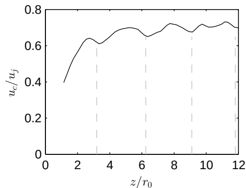
FIGURE 3.13 – Vitesse de convection des structures turbulentes le long de la couche de mélange du jet libre simulé. Les pointillés gris indiquent les fins de cellules du réseau de cellules de chocs.
