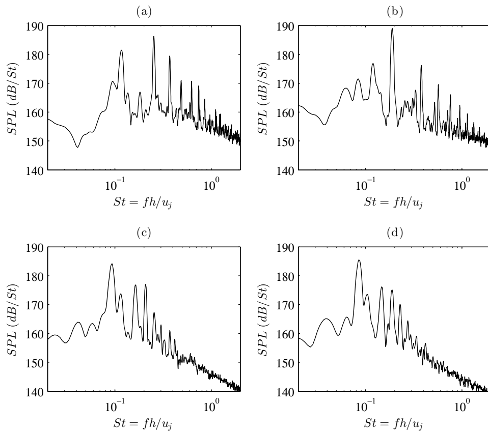
FIGURE 4.12 – Spectres acoustiques (SPL) en x = 0 et y = 1.5h en fonction du nombre de Strouhal pour (a) JetpL3, (b) JetpL5, (c) JetpL8 et (d) JetpL9.
