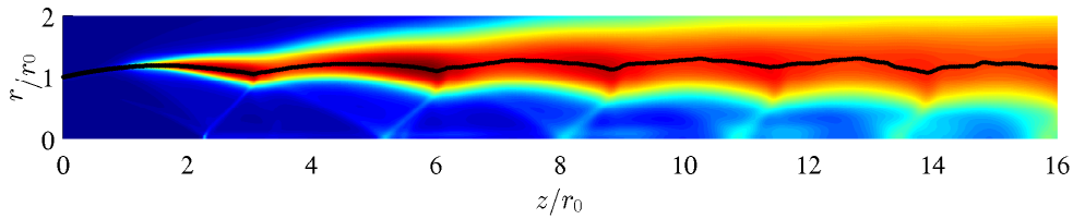
FIGURE 3.12 – Champ de vitesse rms totale du jet libre simulé. L'échelle de couleur varie de 0 à 100 m.s -1 . La ligne noire indique la position radiale de la valeur maximale du champ.
