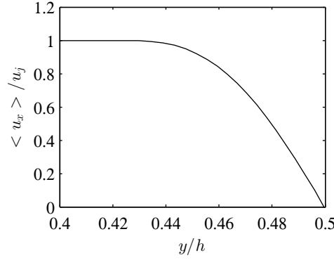
FIGURE 4.2 – Profil de vitesse moyenne axiale en sortie de la buse.
