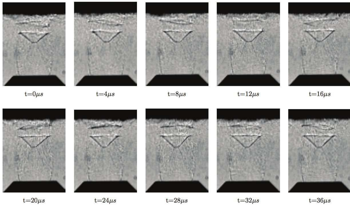
FIGURE 1.20 – Images shadowgraph montrant le cycle complet d'un mode d'impact hélicoïdal pour un jet rond impactant une paroi située en 2D avec un angle normal, et pour un taux de détente de 4, d'après Risborg et Soria [116].
