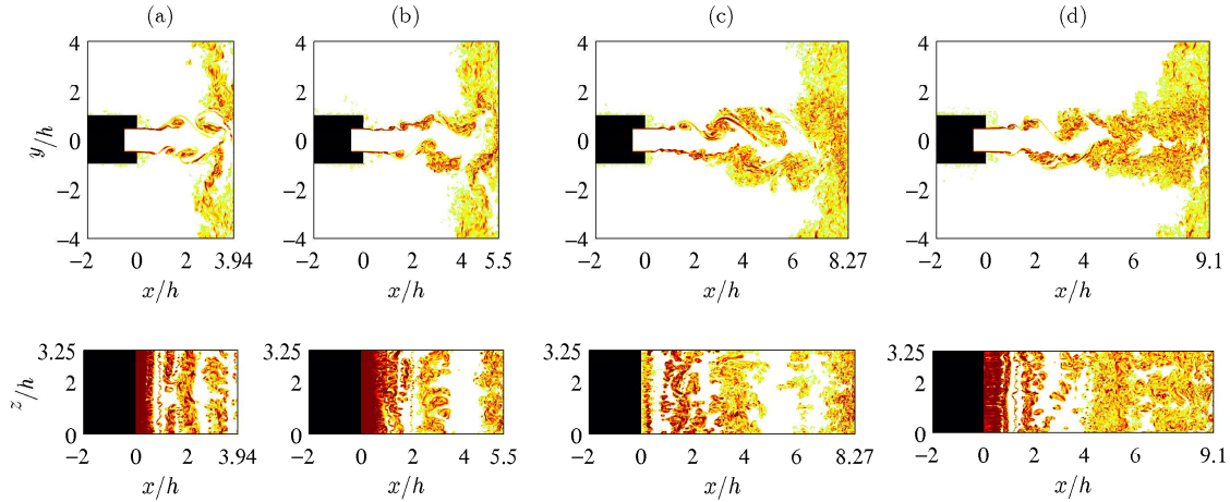
FIGURE 4.5 – Représentations instantanées de la norme de la vorticité |\omega| dans les plans (x, y) et (x, z) le long de la couche de mélange y = h/2 pour (a) JetpL3, (b) JetpL5, (c) JetpL8 et (d) JetpL9. L'échelle de couleur varie pour des valeurs de 0 à 10u_j/h . La buse est en noir.
