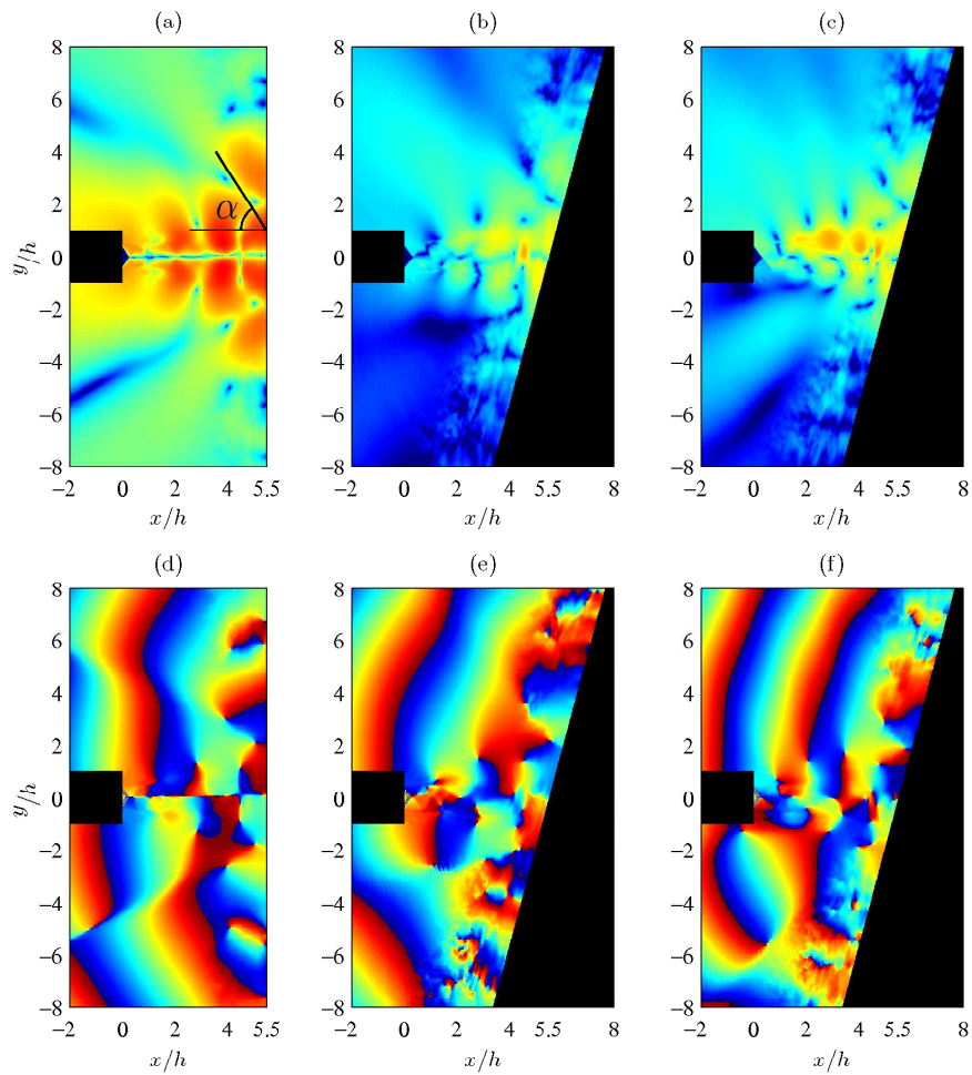
FIGURE 4.34 – Champs d’amplitude (haut) et de phase (bas) obtenus pour les fréquences tonales (a) et (d) de JetpL5 à St_h = 0.19 , (b) et (e) de JetLp5-75d à St_h = 0.19 , et (c) et (f) de JetLp5-75d à St_h = 0.25 .
