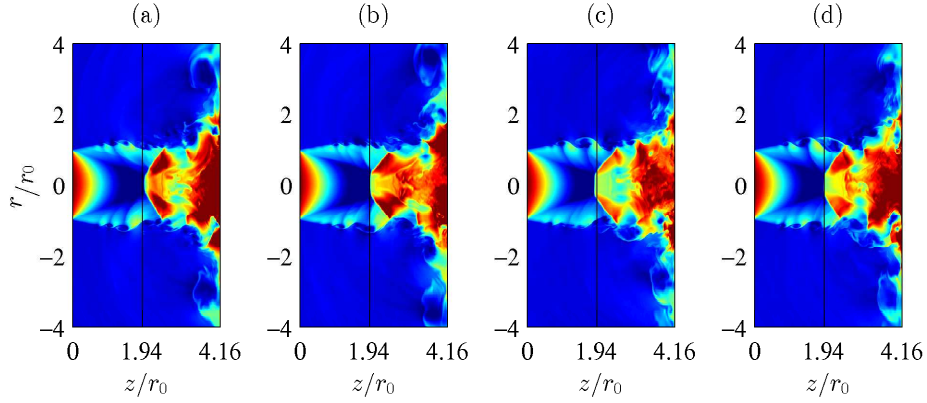
FIGURE 3.42 – Représentations instantanées de la masse volumique dans le plan (z, r) à (a) un temps T_0 , (b) T_0 + T_2/4 , (c) T_0 + T_2/2 et (d) T_0 + 3T_2/4 , où T_2 est la période correspondant à la fréquence tonale St_2 = 0.505 .
