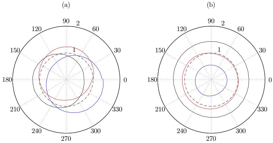
FIGURE 3.38 – Représentation polaire de la pression fluctuante sur le cercle de coordonnées z = 0 et r = 2r_0 pour JetL4, (a) filtrée autour de St_1 = 0.375 à trois instants séparés de T_1/3 et (b) filtrée autour de St_2 = 0.505 à trois instants séparés de T_2/4 ; — — — cercle de rayon unitaire.
