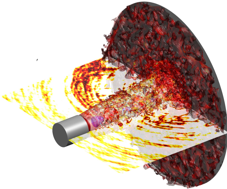
FIGURE 3.24 – Visualisation 3-D du jet JetL9. Les isosurfaces en mauve et rouge correspondent aux valeurs 0.8 et 2.5 \text{ kg.m}^{-3} . Les isosurfaces associées à la valeur de 1.25 \text{ kg.m}^{-3} sont également représentées et sont colorées par le nombre de Mach local. Le champ de pression fluctuante dans le plan \theta = 0 degré est aussi montré. La buse et la paroi sont en gris.
