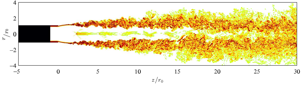
FIGURE 3.4 – Repr  sentation instantan  e dans le plan (z, r) de la norme de la vorticit   |\omega| pour le jet libre. L'  chelle de couleur varie pour des valeurs de 0    10u_j/D_j . La buse est en noir.
