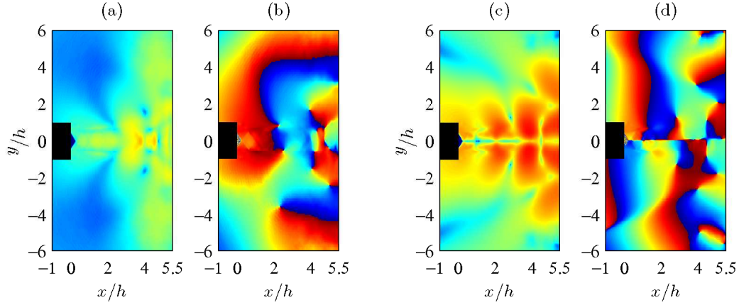
FIGURE 4.19 – Champs d'amplitude et de phase obtenus pour les deux fréquences tonales de JetpL5 (a) et (b) à St_1 = 0.12 , et (c) et (d) à St_2 = 0.19 .
