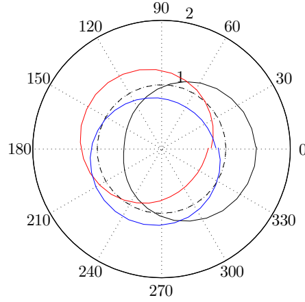
FIGURE 3.17 – Représentation polaire de la pression fluctuante filtrée autour de St = 0.305 en fonction de la direction azimutale, sur le cercle z = 0 et r = 2r_0 , à trois instants séparés de T/3 ; — — — cercle de rayon unitaire.
