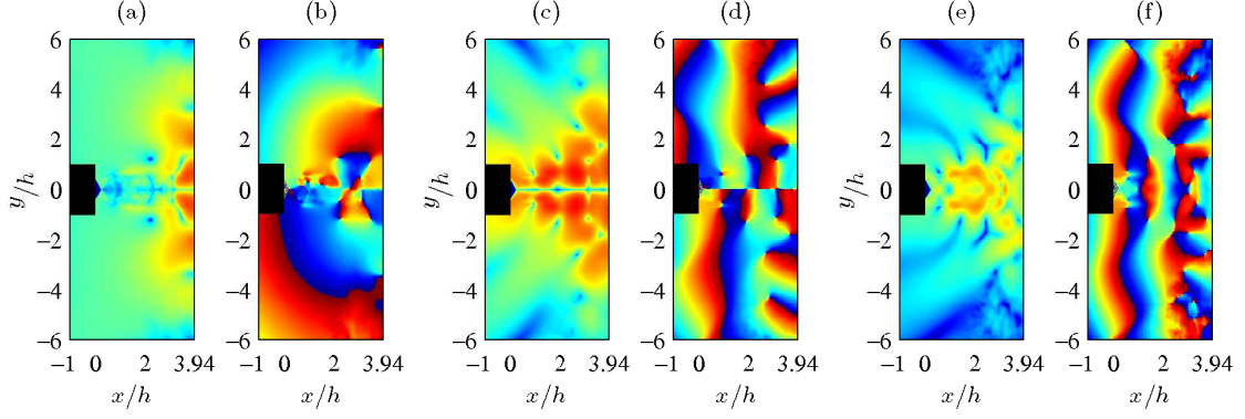
FIGURE 4.17 – Champs d’amplitude et de phase obtenus pour les trois fréquences tonales de JetpL3 (a) et (b) à St_1 = 0.115 , (c) et (d) à St_2 = 0.255 , et (e) et (f) à St_3 = 0.37 .
