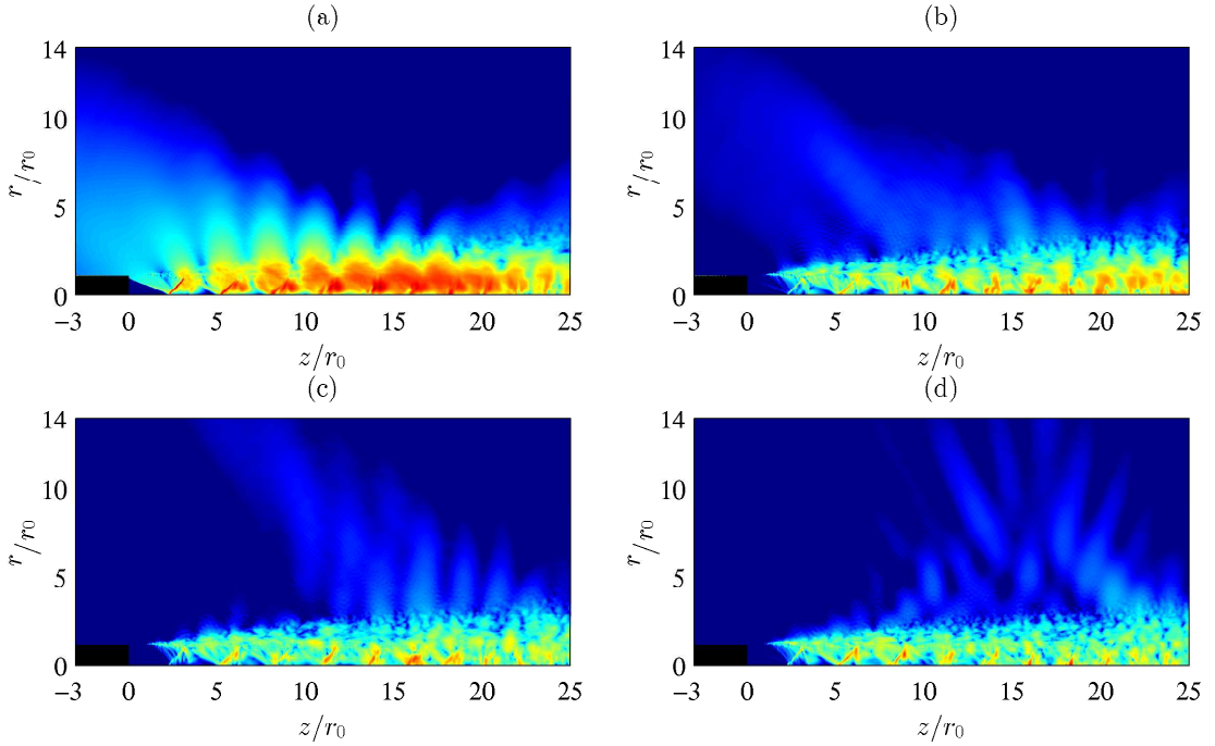
FIGURE 3.20 – Champs d'amplitude dans le plan (z, r) obtenus pour les fréquences (a) St = 0.305 , (b) St = 0.40 , (c) St = 0.50 et (d) St = 0.60 .
