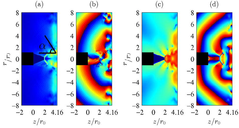
FIGURE 3.37 – Champs d’amplitude et de phase obtenus pour les deux fréquences tonales de JetL4 (a) et (b) à St_1 = 0.375 , et (c) et (d) à St_2 = 0.505 .
