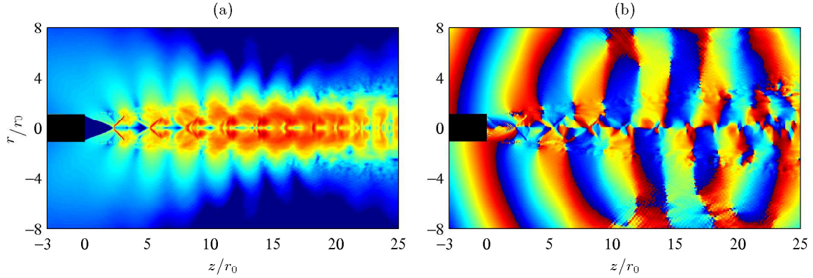
FIGURE 3.15 – Champs d’amplitude (a) et de phase (b) dans le plan (z, r) obtenus pour la fréquence tonale St = 0.305 .
