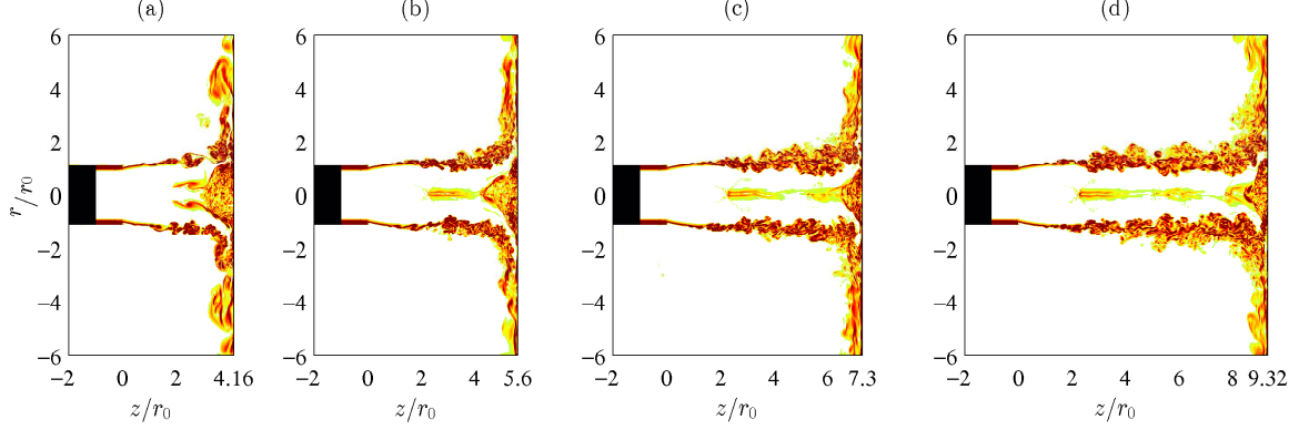
FIGURE 3.25 – Repr sentations instantan es de la norme de la vorticit  |\omega| dans le plan (z, r) pour (a) JetL4, (b) JetL5, (c) JetL7 et (d) JetL9. L' chelle de couleur varie pour des valeurs de 0   10u_j/D_j . La buse est en noir.
