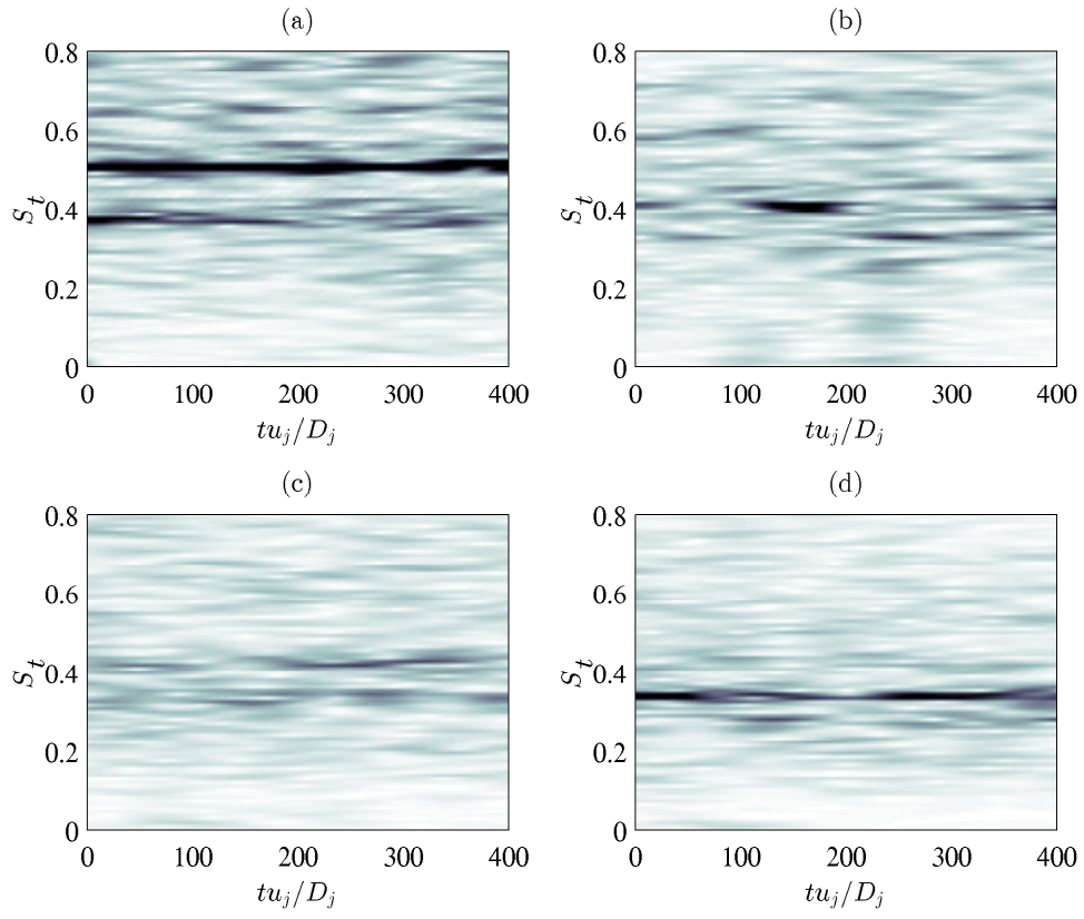
FIGURE 3.46 – Spectres acoustiques au point de coordonnées r = 2r_0 et z = 0 en fonction du temps et du nombre de Strouhal pour (a) JetL4, (b) JetL5, (c) JetL7 et (d) JetL9.
