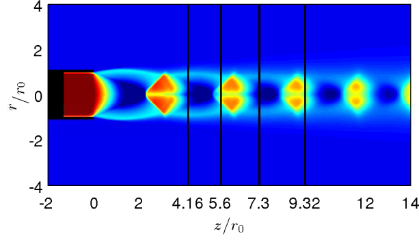
FIGURE 3.21 – Champ moyen de masse volumique obtenu dans le plan (z, r) pour le jet libre. L'échelle de couleur varie pour des valeurs de 1 à 3 \text{ kg.m}^{-3} . Les lignes noires indiquent les positions des parois pour les quatre jets impactant une paroi.
