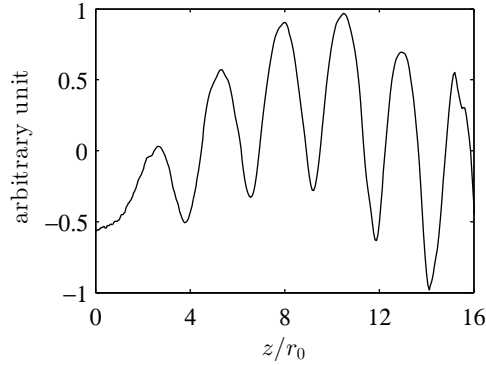
FIGURE 3.16 – Amplitude du spectre à la fréquence tonale St = 0.305 le long de la ligne r = 3r_0 .
