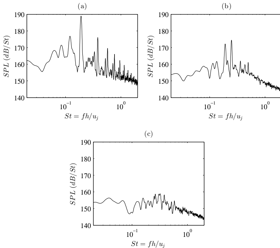
FIGURE 4.31 – Spectres acoustiques (SPL) en x = 0 et y = 1.5h en fonction du nombre de Strouhal pour (a) JetpL5, (b) JetpL5-75d et (c) JetpL5-60d.
