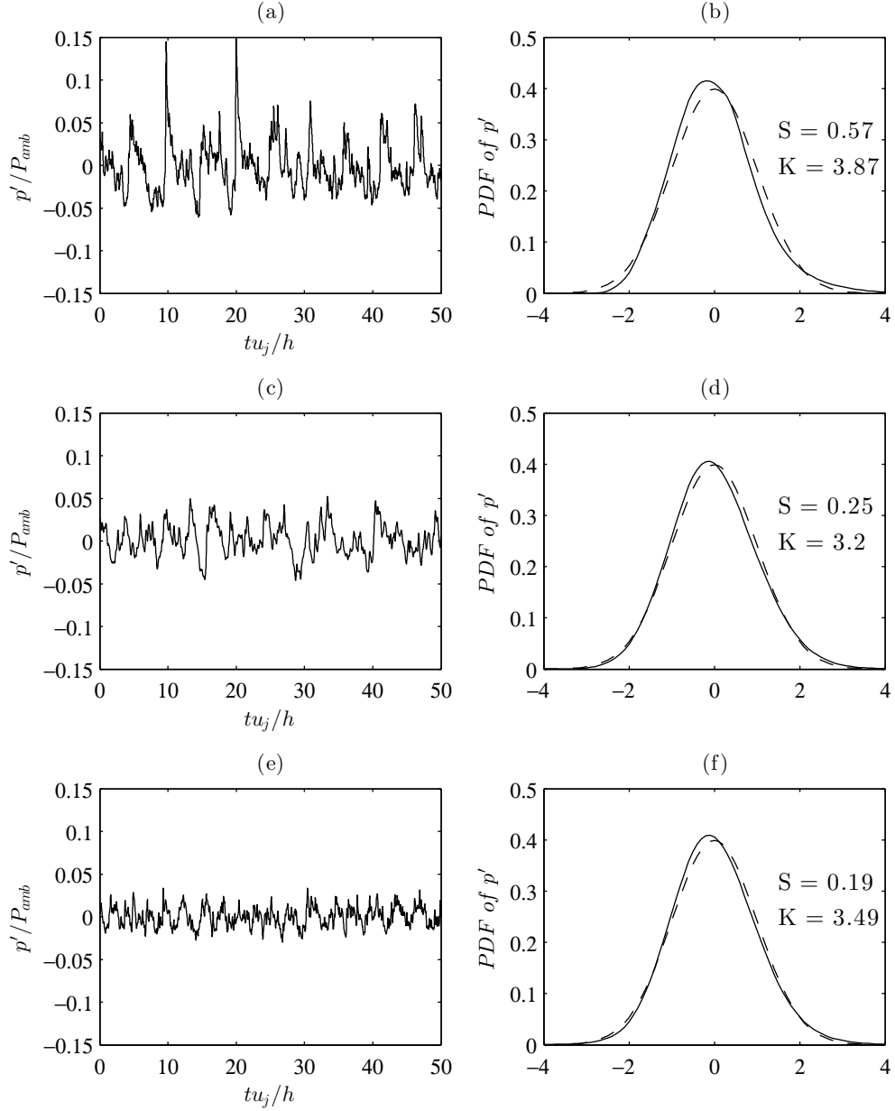
FIGURE 4.33 – Evolution temporelle de la pression fluctuante en x = 0 et y = 8.5h pour (a) JetpL5, (c) JetpL5-75d et (e) JetpL5-60d; densité de probabilité — de la pression fluctuante et — — — d'une distribution gaussienne pour (b) JetpL5, (d) JetpL5-75d et (f) JetpL5-60d.
