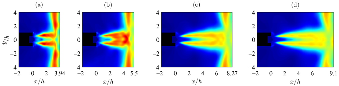
FIGURE 4.9 – Champs rms de la vitesse latérale dans le plan (x, y) pour (a) JetpL3, (b) JetpL5, (c) JetpL8 et (d) JetpL9. L'échelle de couleur varie pour des valeurs de 0 à 100 m.s -1 . La buse est en noir.
