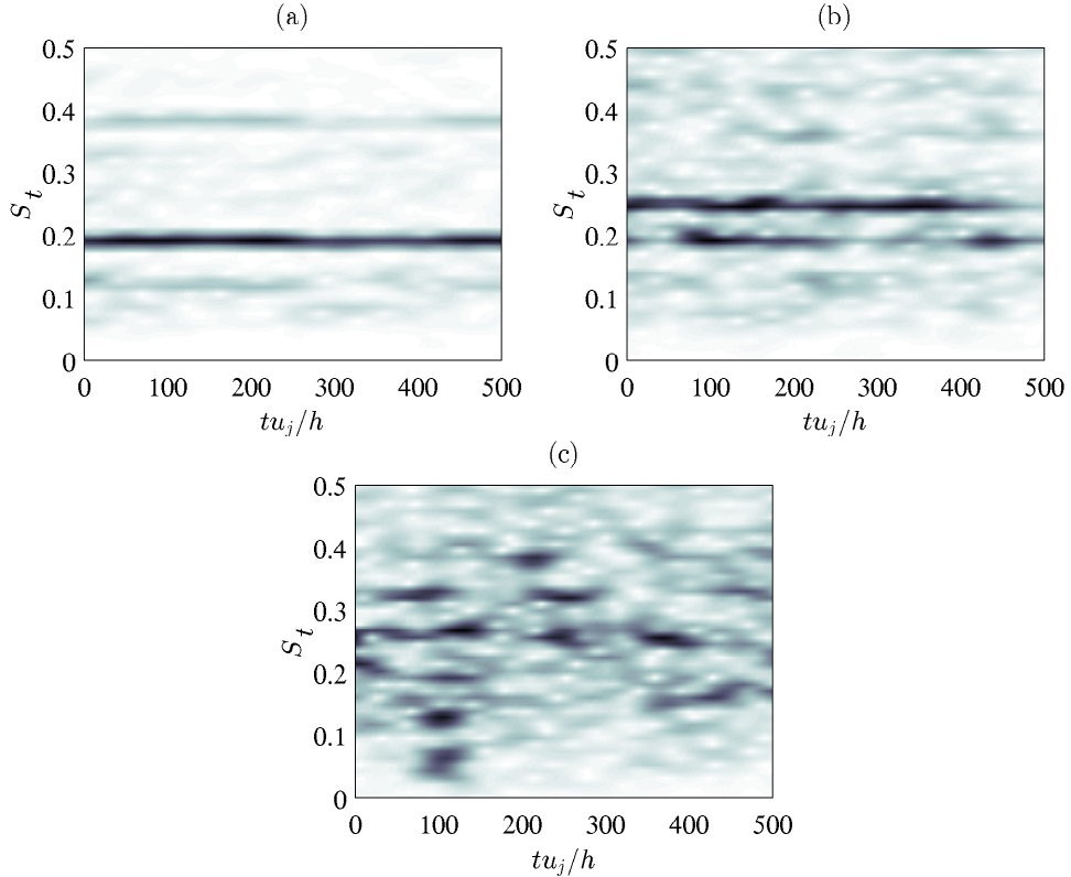
FIGURE 4.35 – Spectres acoustiques au point de coordonnées x = 0 et y = 1.5h en fonction du temps et du nombre de Strouhal pour (a) JetpL5, (b) JetpL5-75d et (c) JetpL5-60d.
