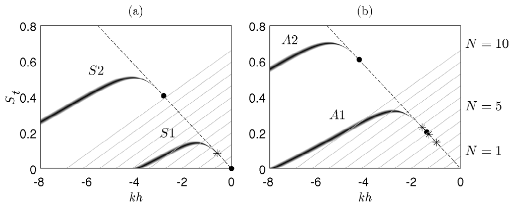
FIGURE 4.24 – — Représentation des relations de dispersion des modes acoustiques neutres (a) symétriques et (b) antisymétriques d’un jet plan supersonique idéalement détendu avec \mathcal{M}_j = 1.28 et h = 2mm ; • limites basses des modes et --- k = -\omega/a_0 ; — condition d’existence d’une onde stationnaire aérodynamique acoustique pour une distance des lèvres de la buse à la paroi de L = 9.1h ; * fréquences tonales pour L = 9.1h .
