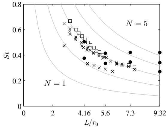
FIGURE 3.36 – Nombres de Strouhal des fréquences tonales obtenues pour • les jets simulés, \square expérimentalement par Henderson et al. [59] pour des jets aux conditions d'éjections similaires et \times expérimentalement par Henderson [58] pour des jets sous-détendus à des nombres de Mach parfaitement détendus de 1.52, 1.58 et 1.64; — valeurs prédites par la relation (3.20).
