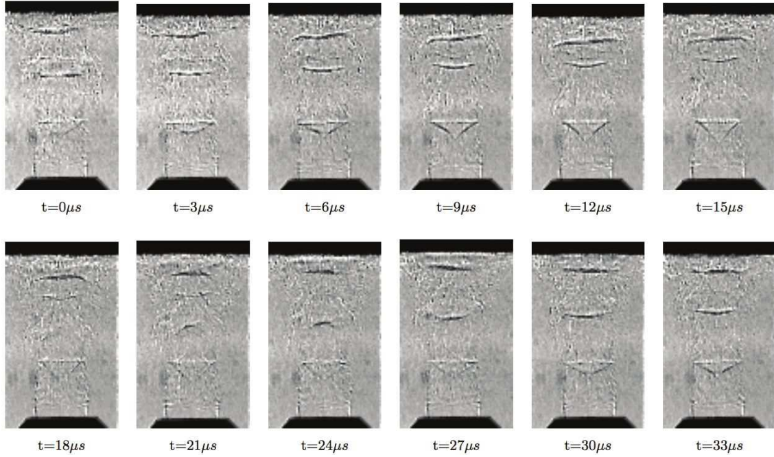
FIGURE 1.21 – Images shadowgraph montrant le cycle complet d'un mode de battement axial pour un jet rond impactant une paroi située en 3D avec un angle de 90 degrés, et pour un taux de détente de 4, d'après Risborg et Soria [116].
