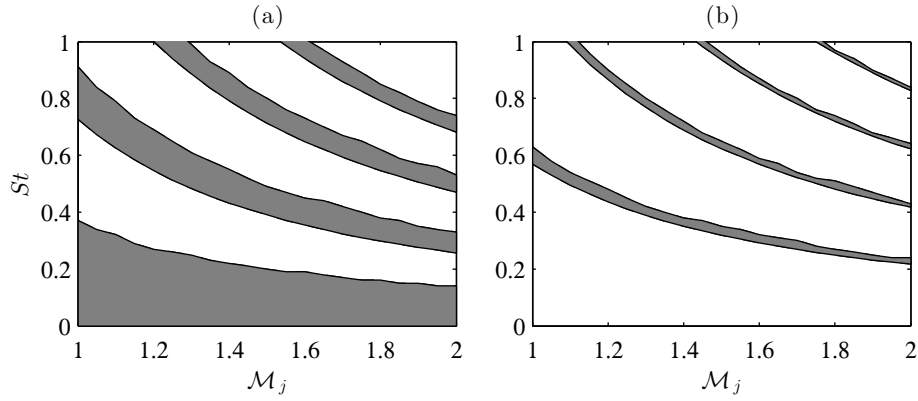
FIGURE 1.18 – Plages de fréquences envisageables pour les quatre premiers modes (a) axisymétriques et (b) hélicoïdaux en fonction du nombre de Mach du jet adapté équivalent et du nombre de Strouhal.
