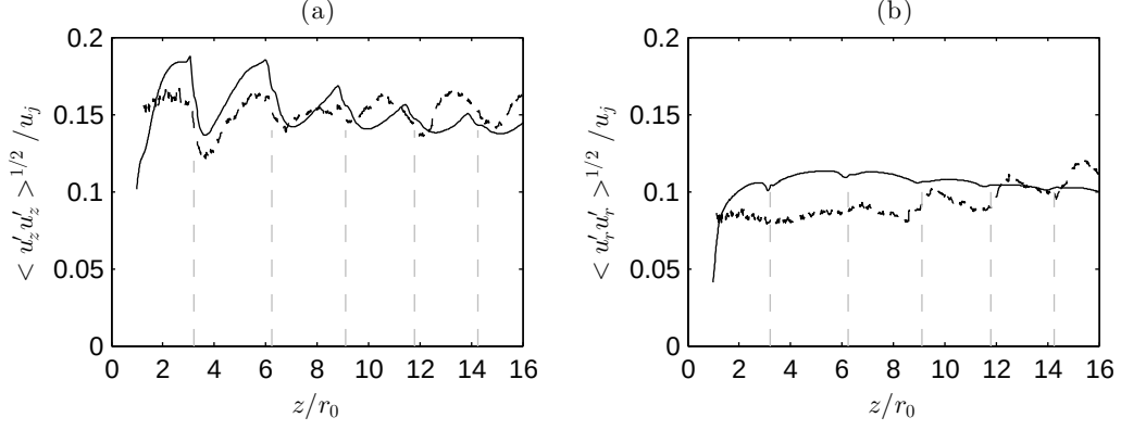
FIGURE 3.11 – Evolution de la valeur maximale de la vitesse rms (a) axiale et (b) radiale le long de la couche de mélange en fonction de la distance axiale; — pour le jet simulé; — — — résultats PIV de André et al. [3]. Les pointillés gris indiquent les fins de cellules du réseau de cellules de chocs dans la LES.
