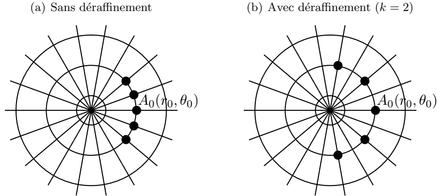
FIGURE 2.6 – Support de la différenciation spatiale azimutale en r = 2\Delta r pour un schéma centré sur 5 points (a) sans déraffinement et (b) avec un déraffinement caractérisé par k = 2 .
