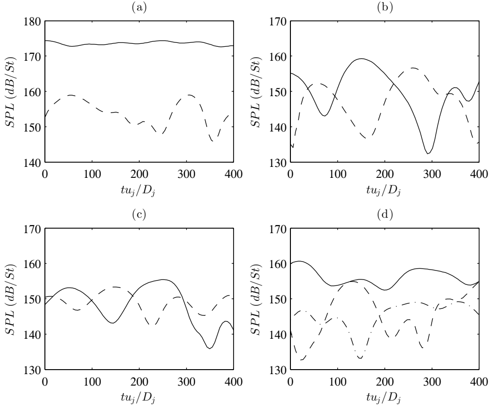
FIGURE 3.47 – Niveaux acoustiques au point de coordonnées r = 2r_0 et z = 0 en fonction du temps pour les fréquences tonales de (a) JetL4 (— — — St_1 = 0.375 et — St_2 = 0.505 ), (b) JetL5 (— — — St_1 = 0.335 et — St_2 = 0.415 ), (c) JetL7 (— — — St_1 = 0.345 et — St_2 = 0.42 ) et (d) JetL9 (— — — St_1 = 0.27 , — St_2 = 0.34 et — · — St_3 = 0.42 ).
