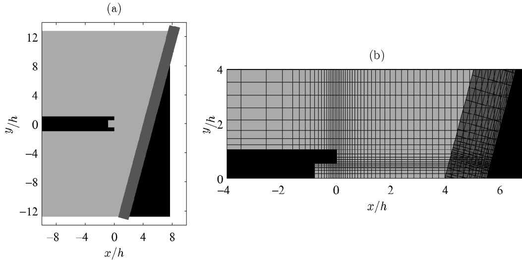
FIGURE 4.1 – Représentation des deux maillages cartésiens à pas variable dans le plan (x, y) dans le cas d'un angle d'impact de 75 degrés; (a) domaine de calcul complet, (b) région limitée à -4 \leq x/h \leq 7 et 0 \leq y/h \leq 4 ; un point sur quinze est montré.
