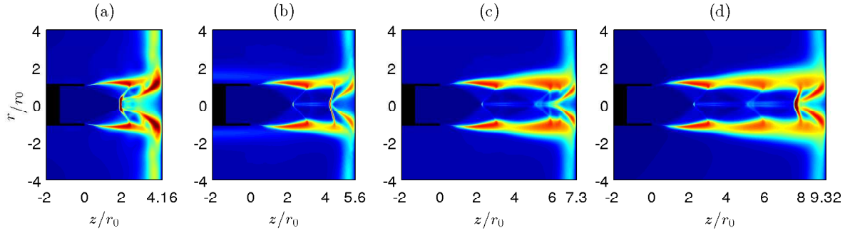
FIGURE 3.30 – Champs rms de la vitesse axiale obtenus dans le plan (z, r) pour (a) JetL4, (b) JetL5, (c) JetL7 et (d) JetL9. L'échelle de couleur varie pour des valeurs de 0 à 100 m.s -1 . La buse est en noir.
