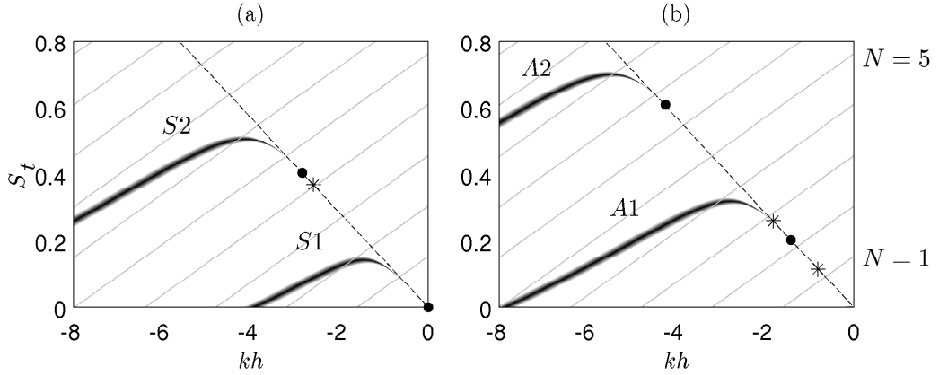
FIGURE 4.18 – — Représentation des relations de dispersion des modes acoustiques neutres (a) symétriques et (b) antisymétriques d’un jet plan supersonique idéalement détendu avec \mathcal{M}_j = 1.28 et h = 2mm ; • limites basses des modes et — — — k = -\omega/a_0 ; — condition d’existence d’une onde stationnaire aérodynamique acoustique pour une distance des lèvres de la buse à la paroi de L = 3.94h ; * fréquences tonales pour L = 3.94h .
