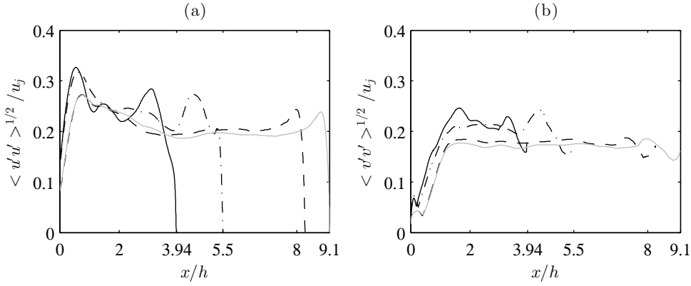
FIGURE 4.10 – Evolution de la valeur maximale de la vitesse rms (a) axiale et (b) latérale le long de la couche de mélange en fonction de la distance axiale pour — JetpL3, - - - JetpL5, - . - JetpL8, et — JetpL9.
