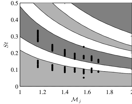
FIGURE 1.14 – Plages de fréquences envisageables pour les deux premiers modes symétriques en gris clair et antisymétriques en gris foncé; • fréquences tonales de la boucle de rétroaction aéroacoustique obtenues expérimentalement par Tam et Norum [143] dans le cas d'un jet froid.
