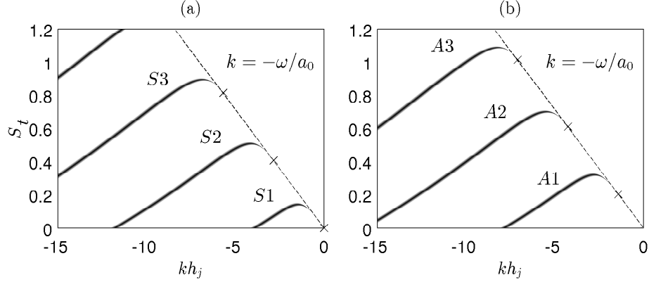
FIGURE 1.13 – Relation de dispersion des modes acoustiques neutres (a) symétriques et (b) antisymétriques d'un jet plan supersonique idéalement détendu avec \mathcal{M}_j = 1.28 et h = 2\text{mm} ; \times limites basses des modes et - - - k = -\omega/a_0 .
