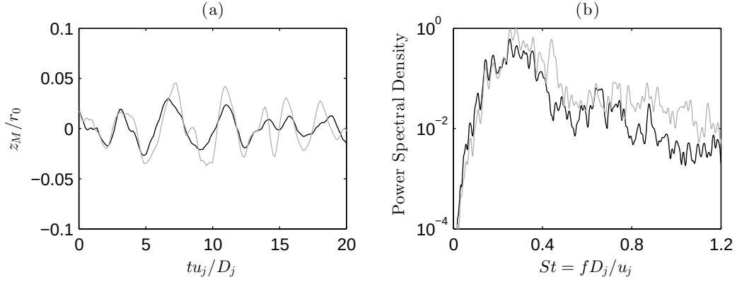
FIGURE 3.44 – (a) Position axiale du choc z_M au cours du temps et (b) densité spectrale de puissance de cette position pour jetL5; — résultats pour le disque de Mach sur l’axe du jet, et — résultats pour le disque de Mach sur la ligne r = 0.7r_0 . L’échelle de la densité spectrale de puissance est arbitraire.
