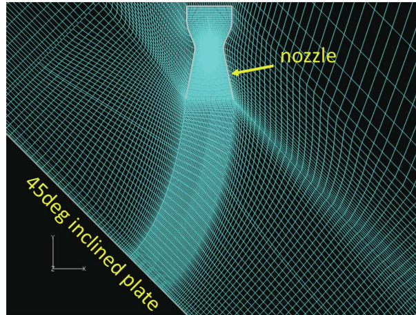
FIGURE 2.8 – Maillage structuré curviligne 2-D utilisé par Nonomura et al. [96] pour étudier l'onde de souffle produite par un jet supersonique impactant une paroi avec un angle de 45 degrés.
