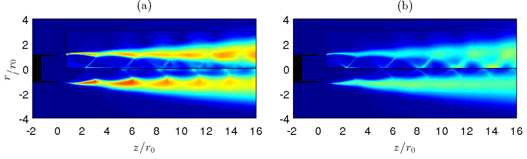
FIGURE 3.10 – Champs de vitesse rms (a) axiale et (b) radiale dans le plan (z, r) . L'échelle de couleur varie pour des valeurs de 0 à 100 \text{m.s}^{-1} . Les résultats PIV de André et al. [3] pour un jet supersonique sous-détendus ( \mathcal{M}_j = 1.5 et \mathcal{M}_e = 1 ) sont représentés dans les rectangles noirs.
