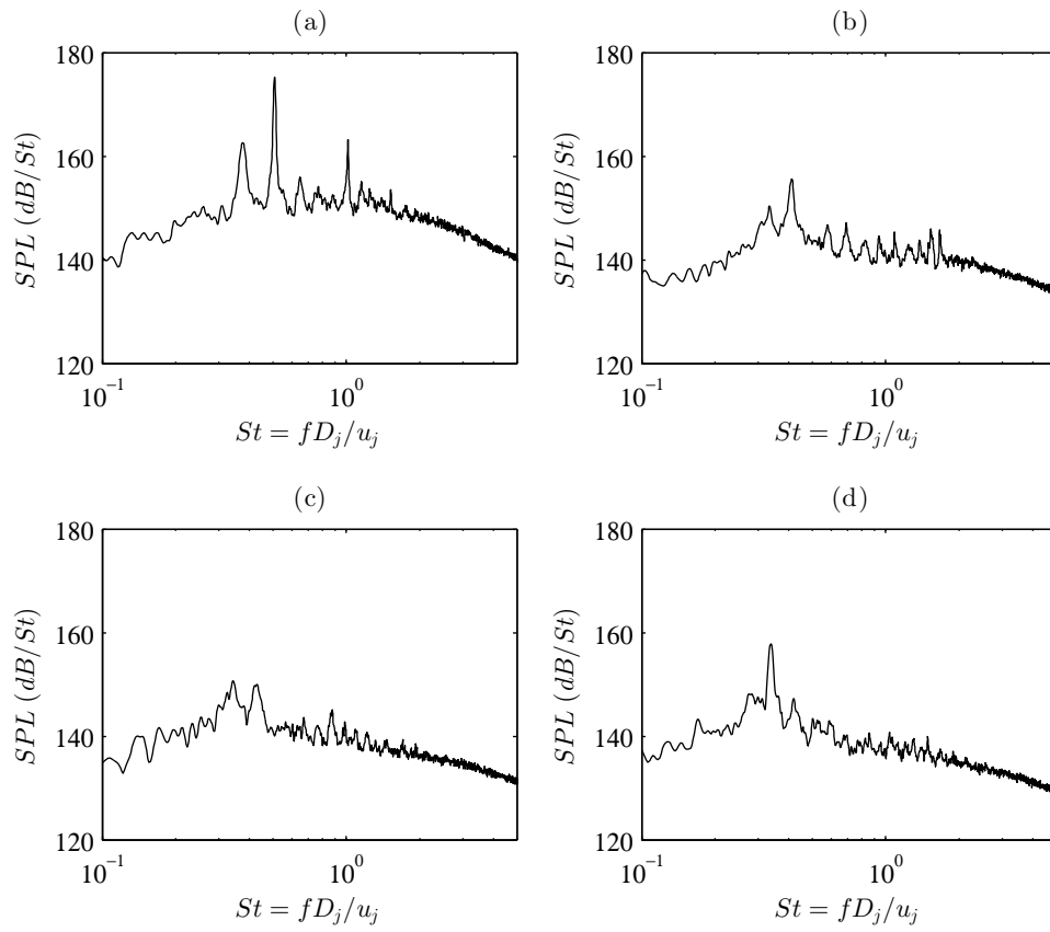
FIGURE 3.35 – Spectres acoustiques (SPL) en r = 2r_0 et z = 0 en fonction du nombre de Strouhal pour (a) JetL4, (b) JetL5, (c) JetL7 et (d) JetL9.
