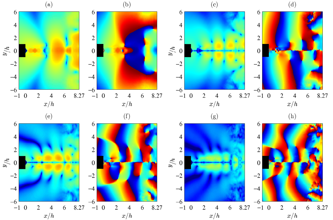
FIGURE 4.21 — Champs d'amplitude et de phase obtenus pour les quatre fréquences tonales de JetpL8 (a) et (b) à St_1 = 0.092 , (c) et (d) à St_2 = 0.165 , (e) et (f) à St_3 = 0.21 , et (g) et (h) à St_4 = 0.255 .
