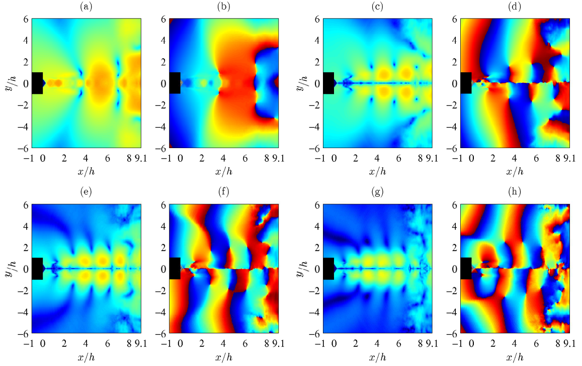
FIGURE 4.23 – Champs d’amplitude et de phase obtenus pour les quatre fréquences tonales de JetpL9 (a) et (b) à St_1 = 0.085 , (c) et (d) à St_2 = 0.145 , (e) et (f) à St_3 = 0.19 , et (g) et (h) à St_4 = 0.23 .
