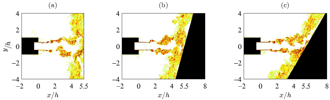
FIGURE 4.26 – Représentations instantanées dans le plan (x, y) de la norme de la vorticité |\omega| pour (a) JetpL5, (b) JetpL5-75d et (c) JetpL5-60d. L'échelle de couleur varie pour des valeurs de 0 à 10u_e/h . La buse et la paroi sont en noir.
