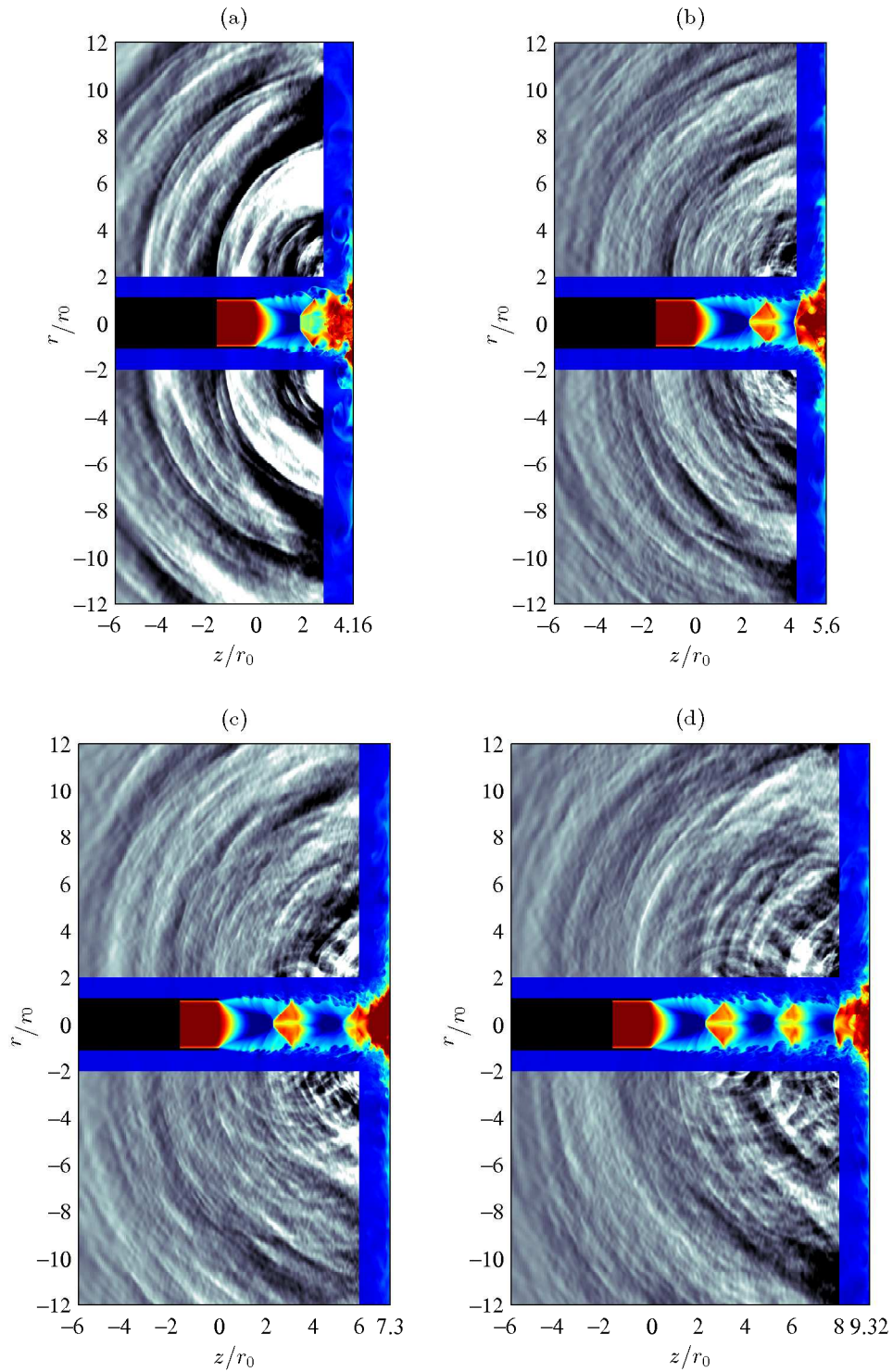
FIGURE 3.26 – Représentations instantanées dans le plan (z, r) de la masse volumique dans les régions proches de l'axe du jet et de la paroi, et de la pression fluctuante pour (a) JetL4, (b) JetL5, (c) JetL7 et (d) JetL9. Les échelles de couleur varient pour des valeurs de 1 à 3 kg.m -3 pour la masse volumique et de -2000 à 2000 Pa pour la pression fluctuante. La buse est en noir.
