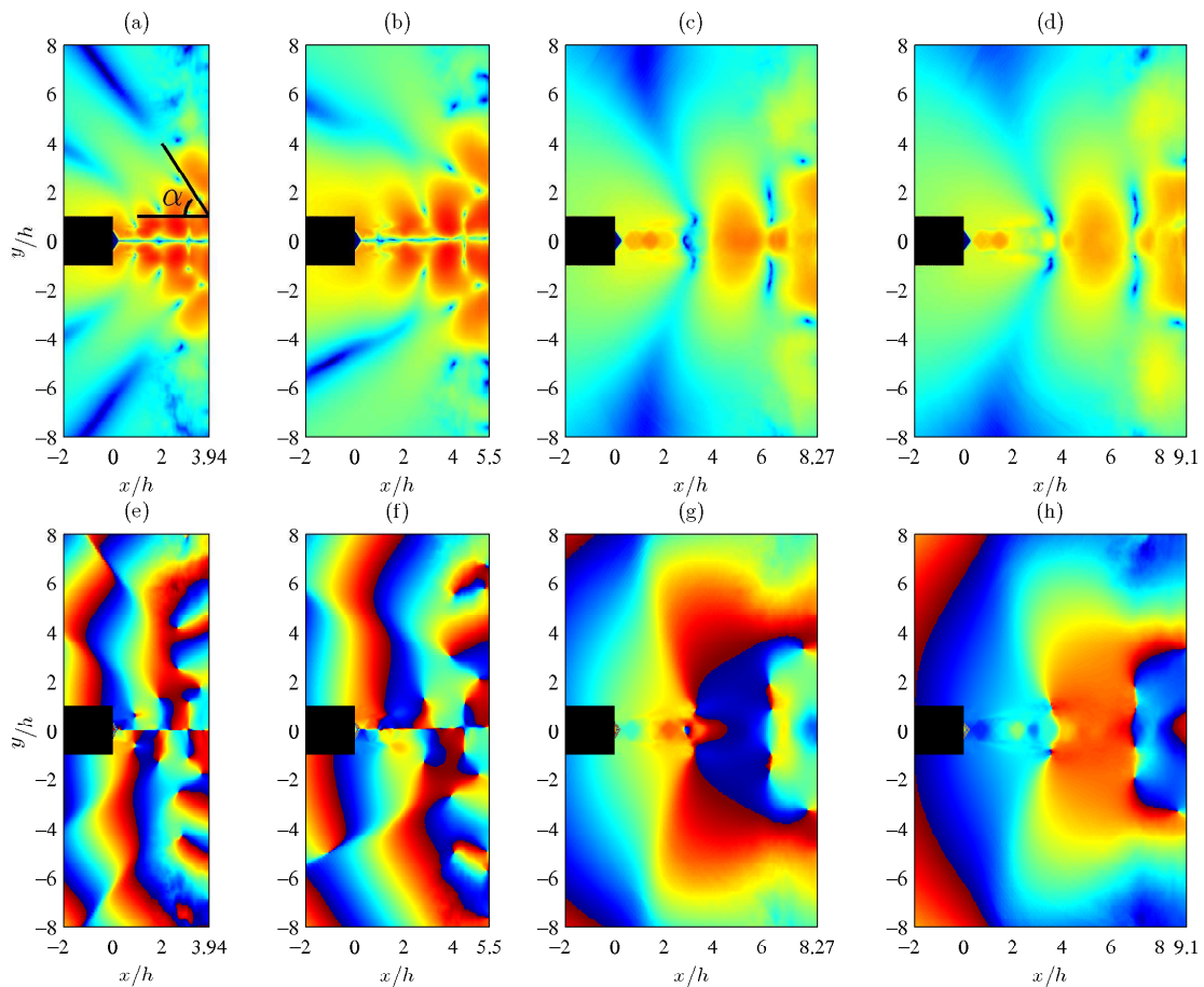
FIGURE 4.15 – Champs d'amplitude (haut) et de phase (bas) obtenus pour les fréquences tonales dominantes de (a) et (e) JetpL3 ( St = 0.255 ), (b) et (f) JetpL5 ( St = 0.19 ), (c) et (g) JetpL8 ( St = 0.092 ), et (d) et (h) JetpL9 ( St = 0.085 ).
