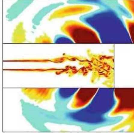
FIGURE 1.3 – Représentation instantanée de la vorticit  et de la pression fluctuante obtenue pour un jet subsonique avec un nombre de Mach de 0.9 et un nombre de Reynolds de 1700 par simulation des grandes  chelles [17].
