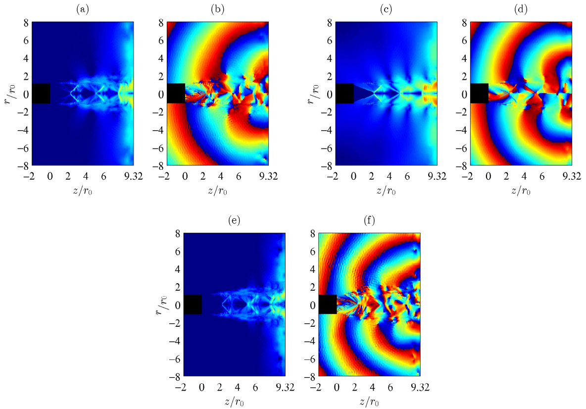
FIGURE 3.41 – Champs d'amplitude et de phase obtenus pour les trois fréquences tonales de JetL9 (a) et (b) à St_1 = 0.27 , (c) et (d) à St_2 = 0.34 , et (e) et (f) à St_3 = 0.42 .
