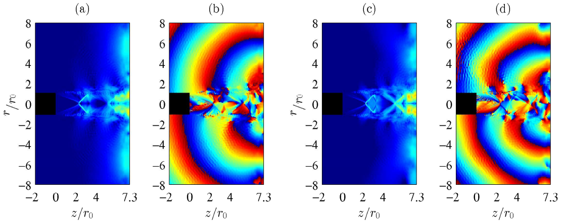
FIGURE 3.40 – Champs d'amplitude et de phase obtenus pour les deux fréquences tonales de JetL7 (a) et (b) à St_1 = 0.345 , et (c) et (d) à St_2 = 0.42 .
