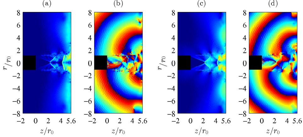
FIGURE 3.39 – Champs d'amplitude et de phase obtenus pour les deux fréquences tonales de JetL5 (a) et (b) à St_1 = 0.335 , et (c) et (d) à St_2 = 0.415 .
