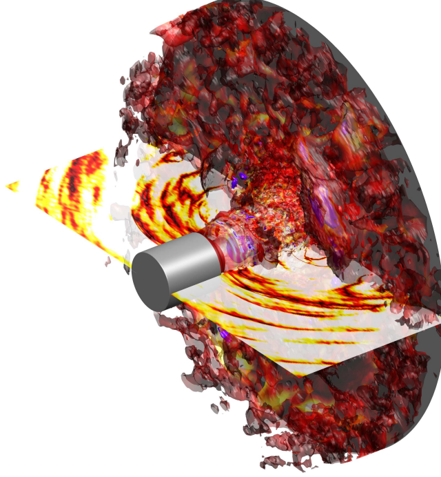
FIGURE 3.23 – Visualisation 3-D du jet JetL4. Les isosurfaces en mauve et rouge correspondent aux valeurs 0.8 et 2.5 \text{ kg.m}^{-3} . Les isosurfaces associées à la valeur de 1.25 \text{ kg.m}^{-3} sont également représentées et sont colorées par le nombre de Mach local. Le champ de pression fluctuante dans le plan \theta = 0 degré est aussi montré. La buse et la paroi sont en gris.
