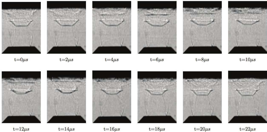
FIGURE 1.19 – Images shadowgraph montrant le cycle complet d'un mode de pulsation axiale pour un jet rond impactant une paroi située en 2D avec un angle normal, et pour un taux de détente de 5, d'après Risborg et Soria [116].
