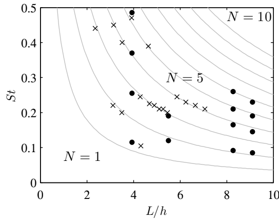
FIGURE 4.14 – Nombre de Strouhal des fréquences tonales obtenues pour • les quatre jets étudiés, × expérimentalement par Thurow et al. [153] pour des jets aux conditions d'éjections similaires. — valeurs prédites par la relation (4.9) avec <u_c> = 0.60u_j .
