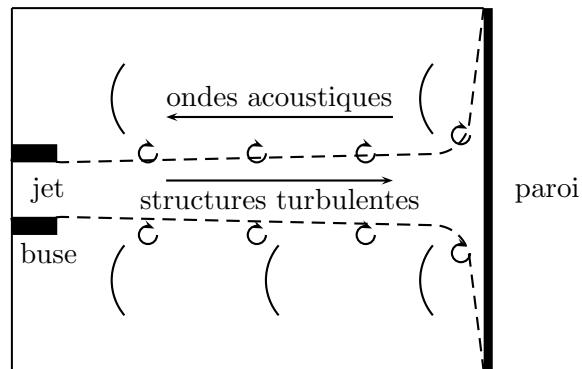
FIGURE 1.8 – Représentation de la boucle de rétroaction aéroacoustique.
