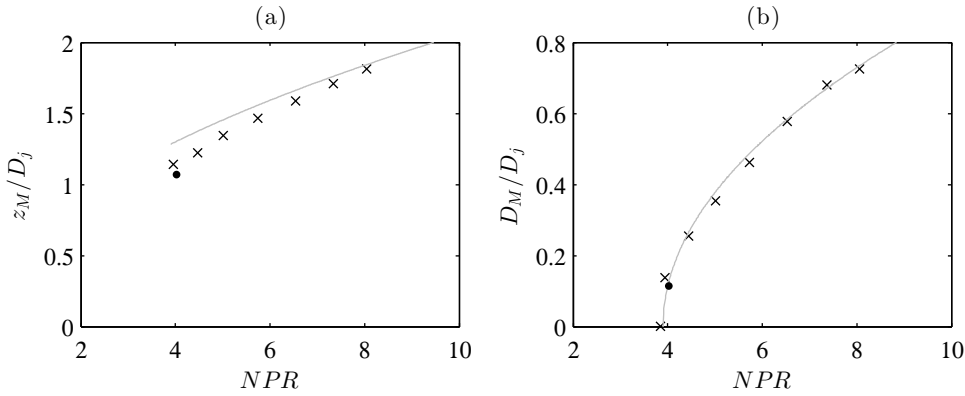
FIGURE 3.9 – (a) Position et (b) diamètre du disque de Mach pour • le jet simulé, × les jets expérimentaux de Addy [1] et — en utilisant les relations (3.12) and (3.13).
