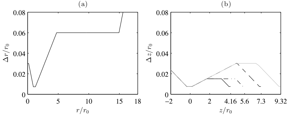
FIGURE 3.22 – Evolution de la taille des mailles dans la direction (a) radiale et (b) axiale pour — JetL4, - · - JetL5, - - - JetL7 et — JetL9.
