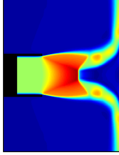
FIGURE 1.9 – Vitesse totale moyenne d'un jet rond supersonique sous-détendu impactant une paroi située à 4 rayons des lèvres de la buse, pour un nombre de Mach parfaitement détendu \mathcal{M}_j = 1.56 , un nombre de Mach d'éjection \mathcal{M}_e = 1 et un nombre de Reynolds de 6 \times 10^4 . Simulation des grandes échelles présentée dans le chapitre 3.
