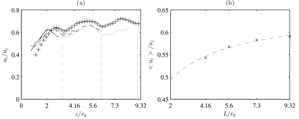
FIGURE 3.34 – (a) Vitesse de convection des structures turbulentes le long des couches de mélange pour — JetL4, —·— JetL5, — — — JetL7, — — — JetL9 et +++ pour le jet libre. Les pointillés gris indiquent les fins des cellules de chocs du jet libre; (b) vitesse moyenne de convection entre la buse et la paroi \times pour les quatre jets impactant et — — — donnée par la relation (3.19), en fonction de la distance L/r_0 .
