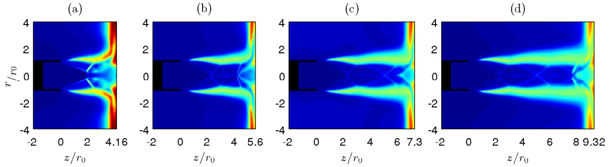
FIGURE 3.31 – Champs rms de la vitesse radiale obtenus dans le plan (z, r) pour (a) JetL4, (b) JetL5, (c) JetL7 et (d) JetL9. L'échelle de couleur varie pour des valeurs de 0 à 100 m.s -1 . La buse est en noir.
