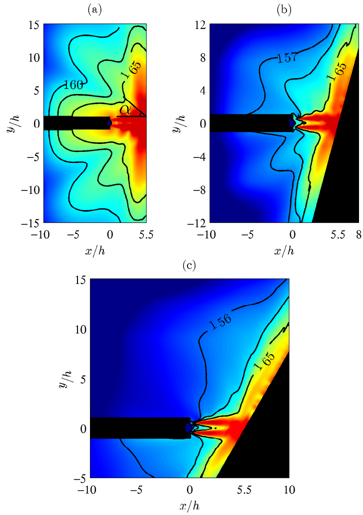
FIGURE 4.29 – Champs de niveaux de puissance acoustique dans le plan (x, y) pour (a) JetpL5, (b) JetpL5-75d et (c) JetpL5-60d. L'échelle de couleur varie pour des valeurs de 150 à 175 dB. La buse et la paroi sont en noir.
