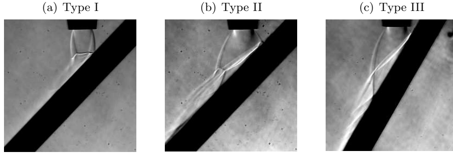
FIGURE 1.10 – (a) Réseau de cellules de type I pour un jet avec un taux de détente de 1.2 et pour une plaque située en L/D = 2 avec un angle de 45 degrés; (b) réseau de cellules de type II pour un jet avec un taux de détente de 4 et pour une plaque située en L/D = 2 avec un angle de 45 degrés; (c) réseau de cellules de type III pour un jet avec un taux de détente de 7 et pour une plaque située en L/D = 2 avec un angle de 30 degrés. Images schlieren de Nakai et al. [92].
