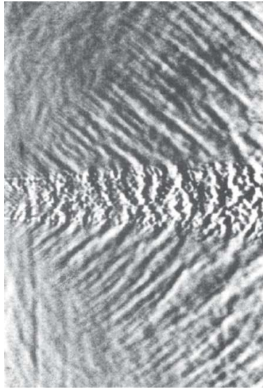
FIGURE 1.4 – Photographie schlieren [99] d'un jet supersonique adapté à un nombre de Mach \mathcal{M}_e = 1.8 .
