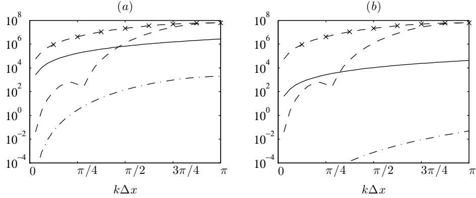
FIGURE 2.11 – Fonctions de transfert associées : — à la dissipation visqueuse, — — — à la dissipation du filtrage explicite centré SFo11p, — · — à la dissipation de l’algorithme d’intégration spatiale RK2 et — * — à la dissipation du filtre de la capture de choc Fopt; (a) pour une taille de maille \Delta x_{min} = 7.5 \times 10^{-6} m et (b) \Delta x_{max} = 6 \times 10^{-5} m de maille dans le domaine de calcul, hors des zones éponges.
