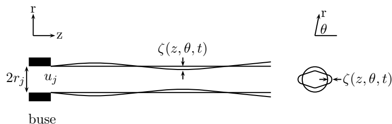
FIGURE 1.16 – Jet supersonique rond entouré par une couche de mélange infiniment mince.
