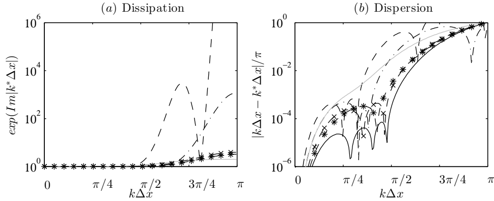
FIGURE 2.1 – Schémas de différences finies centrés de Bogey et Bailly [16] et décentrés de Berland et al. [12]. Erreur de (a) dissipation et de (b) dispersion en fonction du nombre d'onde k\Delta x : — schéma centré FDo11p, — — — schéma décentré FDo010d, — · — schéma décentré FDo19d, — schéma décentré FDo28d, — * — schéma décentré FDo37d et — × — schéma décentré FDo46d.
