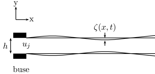
FIGURE 1.12 – Jet supersonique 2-D entouré par deux couches de mélange infiniment minces.
