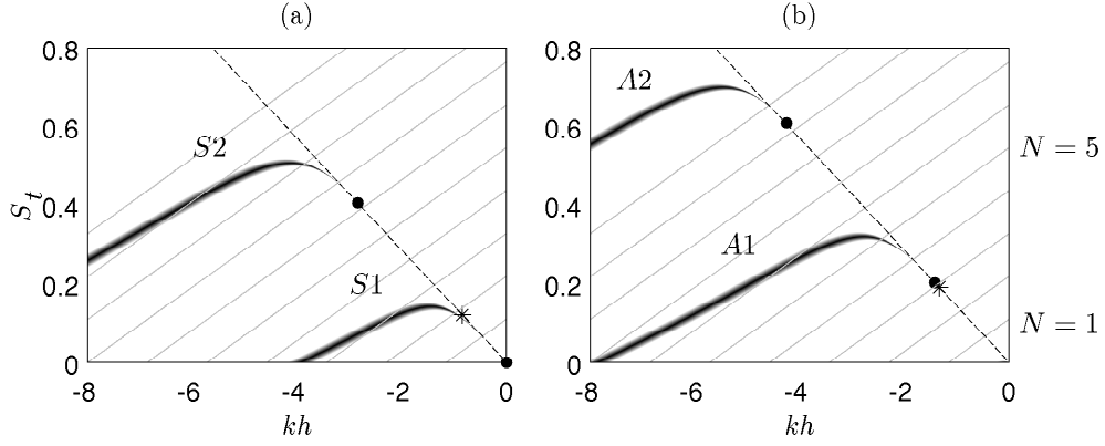
FIGURE 4.20 — Représentation des relations de dispersion des modes acoustiques neutres (a) symétriques et (b) antisymétriques d'un jet plan supersonique idéalement détendu avec \mathcal{M}_j = 1.28 et h = 2mm ; • limites basses des modes et - - - k = -\omega/a_0 ; — condition d'existence d'une onde stationnaire aérodynamique acoustique pour une distance des lèvres de la buse à la paroi de L = 5.5h ; * fréquences tonales pour L = 5.5h .
