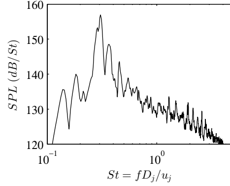
FIGURE 3.14 – Spectre acoustique (SPL) en z = 0 et r = 2r_0 en fonction du nombre de Strouhal du jet libre.
