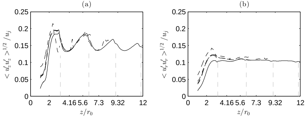
FIGURE 3.32 – Evolution de la valeur maximale de la vitesse rms (a) axiale et (b) radiale le long de la couche de mélange en fonction de la distance axiale; — résultats pour le jet libre et — — — résultats pour les quatre jets impactant. Les pointillés gris indiquent les fins de cellules du réseau de cellules de chocs.
