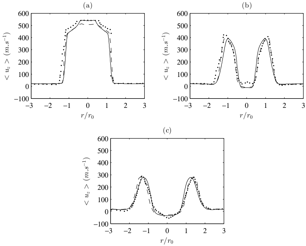
FIGURE 3.29 – Profils de vitesse moyenne axiale en fonction de la direction radiale pour JetL4 à (a) z = 1.5r_0 , (b) z = 3r_0 et (c) z = 3.6r_0 ; — résultats des simulations, - - - résultats expérimentaux de Henderson et al. [59] et • résultats numériques de Dauplain et al. [38].
