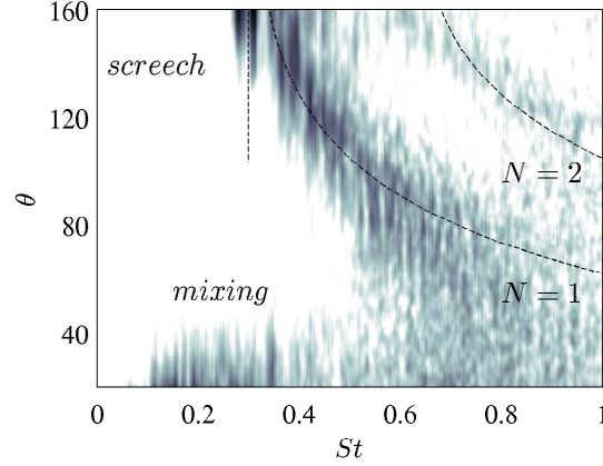
FIGURE 3.19 – Densité spectrale de puissance (PSD pour Power Spectral Density en anglais) des fluctuations de pression sur un cercle dont le centre est situé sur l'axe du jet en z = 15r_0 et dont le rayon vaut 15r_0 , en fonction du nombre de Strouhal et de l'angle d'observation selon la direction aval \theta .
