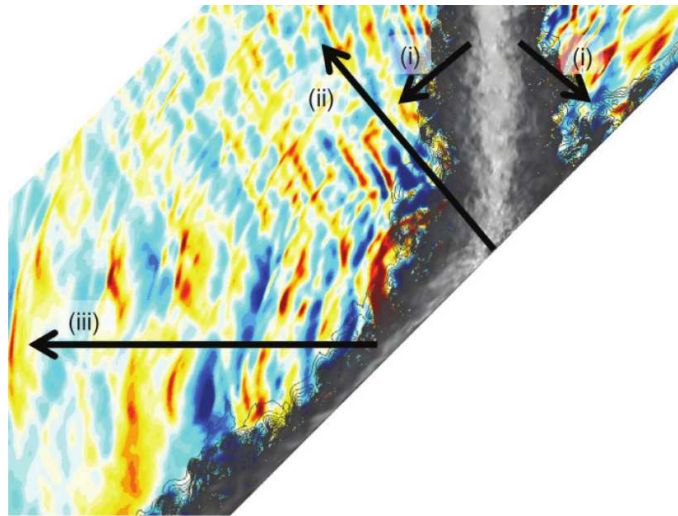
FIGURE 1.11 – Pression fluctuante obtenue par une simulation des grandes échelles d’un jet rond idéalement détendu impactant une paroi avec un angle de 45 degrés, pour un nombre de Mach \mathcal{M}_j = 2 , d’après Nonomura et al. [95]
