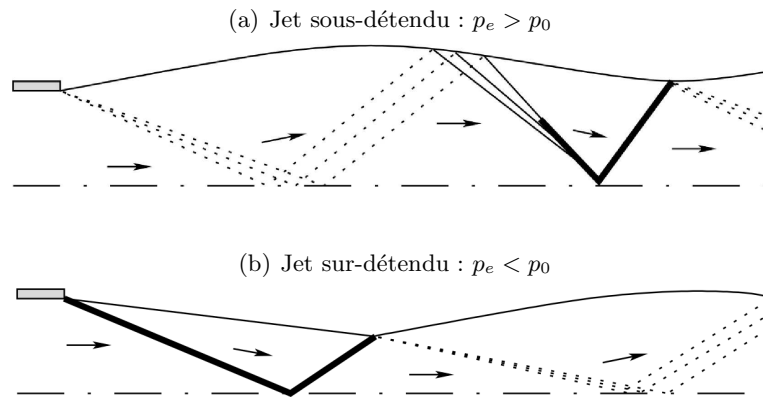
FIGURE 1.2 – Réseau de cellules de chocs pour un jet non-adapté (a) sous-détendu et (b) sur-détendu; — onde de compression, \cdots onde de détente, — choc de compression, ——— axe du jet, \rightarrow direction des lignes de courant et — couche de mélange du jet.
