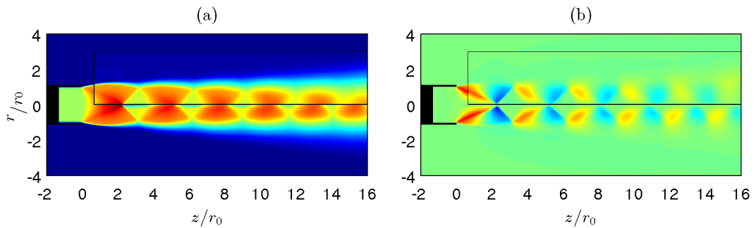
FIGURE 3.6 – Champs moyens dans le plan (z, r) de la vitesse (a) axiale et (b) radiale. Les échelles de couleur varient pour des valeurs de 0 à 600 \text{m.s}^{-1} pour la vitesse axiale et de -150 à 150 \text{m.s}^{-1} pour la vitesse radiale. Les résultats PIV de André et al. [3] pour un jet supersonique sous-détendu ( M_j = 1.5 et M_e = 1 ) sont montrés dans les rectangles noirs.
