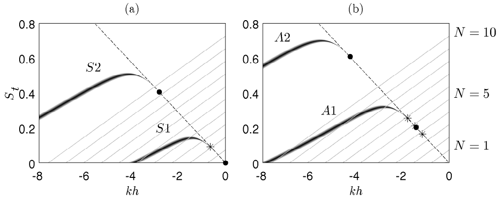
FIGURE 4.22 — Représentation des relations de dispersion des modes acoustiques neutres (a) symétriques et (b) antisymétriques d'un jet plan supersonique idéalement détendu avec \mathcal{M}_j = 1.28 et h = 2mm ; • limites basses des modes et - - - k = -\omega/a_0 ; — condition d'existence d'une onde stationnaire aérodynamique acoustique pour une distance des lèvres de la buse à la paroi de L = 8.27h ; * fréquences tonales pour L = 8.27h .
