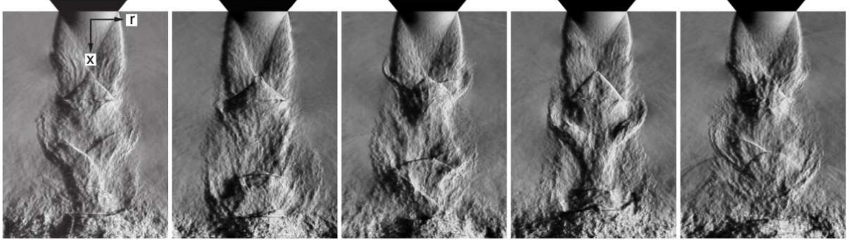
FIGURE 1.7 – Images schlieren d'un jet rond supersonique sous-détendu à M_j = 1.4 , impactant une paroi perpendiculaire située à 4D des lèvres de la buse, d'après Buchmann et al. [25]
