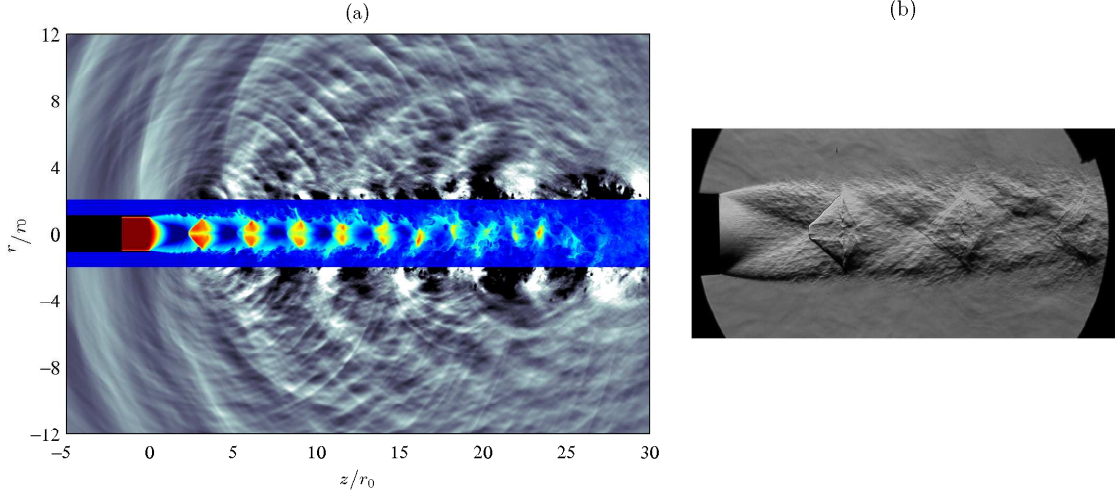
FIGURE 3.5 – (a) Représentation instantanée dans le plan (z, r) de la masse volumique dans la région proche de l'axe et de la pression fluctuante pour le jet libre. Les échelles de couleur varient pour des valeurs de 1 à 3 \text{kg.m}^{-3} pour la densité et de -2000 à 2000 Pa pour la pression fluctuante; (b) photographie schlieren d'un jet supersonique sous-détendu ( M_j = 1.55 et M_e = 1 ) de André et al. [3].
