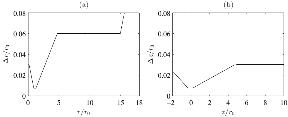
FIGURE 3.2 – Evolutions de la taille des mailles dans les directions (a) radiale et (b) axiale.
