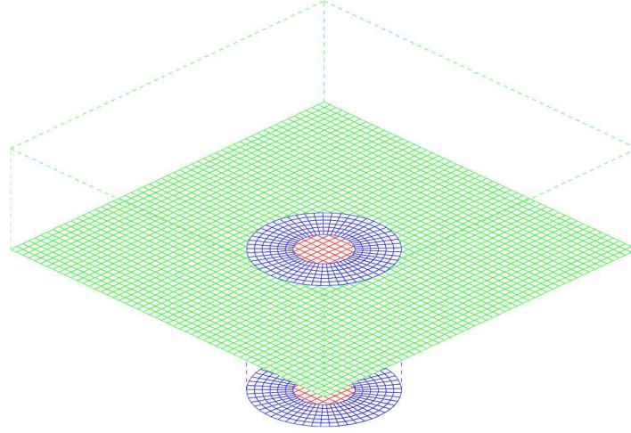
FIGURE 2.9 – Méthode de recouvrement de maillages pour le calcul du bruit rayonné par un écoulement affleurant une cavité cylindrique par Marsden et al. [85]. Le maillage cylindrique bleu permet la discrétisation de la paroi de la cavité cylindrique, le maillage cartésien rouge celle de l'intérieur de la cavité et le maillage cartésien vert celle de la paroi.
