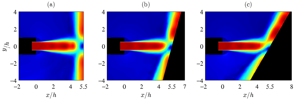
FIGURE 4.28 – Champs moyens de vitesse totale dans le plan (x, y) pour (a) JetpL5, (b) JetpL5-75d et (c) JetpL5-60d. L'échelle de couleur varie pour des valeurs de 0 à 400 m.s -1 . La buse et la paroi sont en noir.
