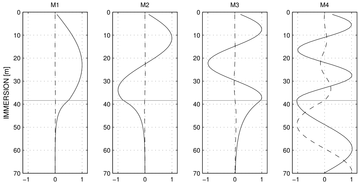
FIG. 2.10 – Fonctions modales des trois modes propres (respectivement M1, M2 et M3) et du mode dissipatif (M4) pour une valeur d'atténuation du son dans le fond de 0.5 dB/λ.
