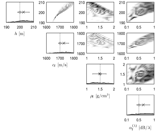
FIG. B.4 – Corrélations entre paramètres (à gauche) et densités marginales a posteriori 1D (à droite en diagonale) et 2D (à droite hors diagonale) pour une antenne verticale située à une distance de 10 km pour une fréquence de 15 Hz.
