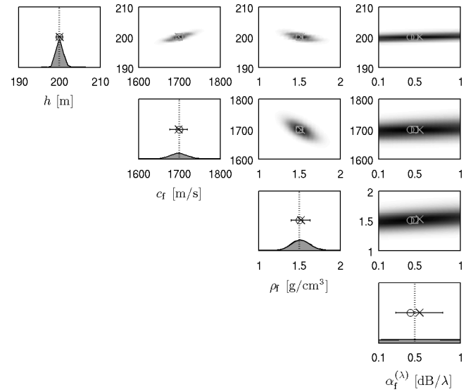
FIG. B.5 – Corrélations entre paramètres (à gauche) et densités marginales a posteriori 1D (à droite en diagonale) et 2D (à droite hors diagonale) pour une antenne verticale située à une distance de 0.5 km pour une fréquence de 25 Hz.
