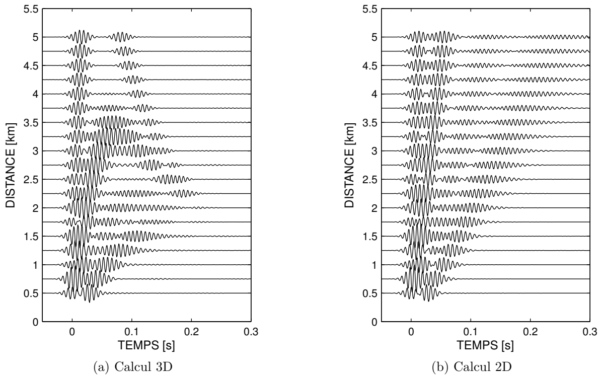
FIG. 2.26 – Prédictions numériques (code 3DWAPE) pour les signaux temporels reçus en fonction de la distance, pour une immersion de récepteur de 20 m. (a) Calcul 3D et (b) calcul 2D. L'immersion de la source est z_S = 10 m).
