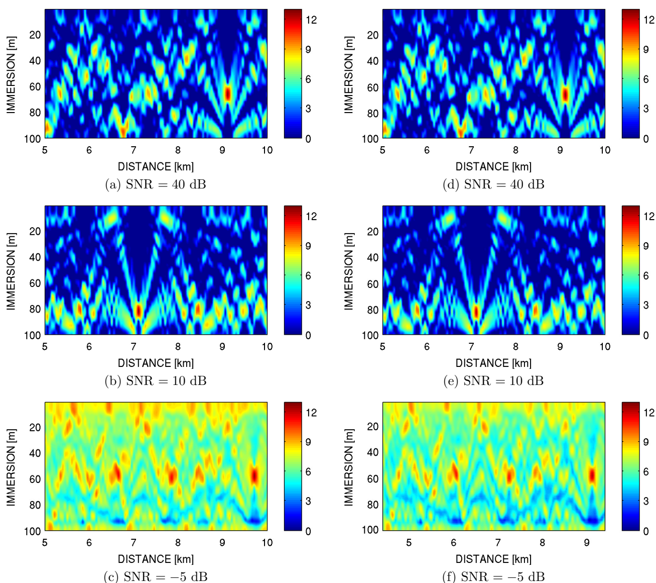
FIG. 1.7 – Localisation de la source pour le cas test COLNOISE avec le code RAM (à gauche) pour un rapport signal-sur-bruit de (a) 40 dB, (b) 10 dB, (c) -5 dB et avec le code 3DWAPE (à droite) pour un rapport signal-sur-bruit de (d) 40 dB, (e) 10 dB, (f) -5 dB
