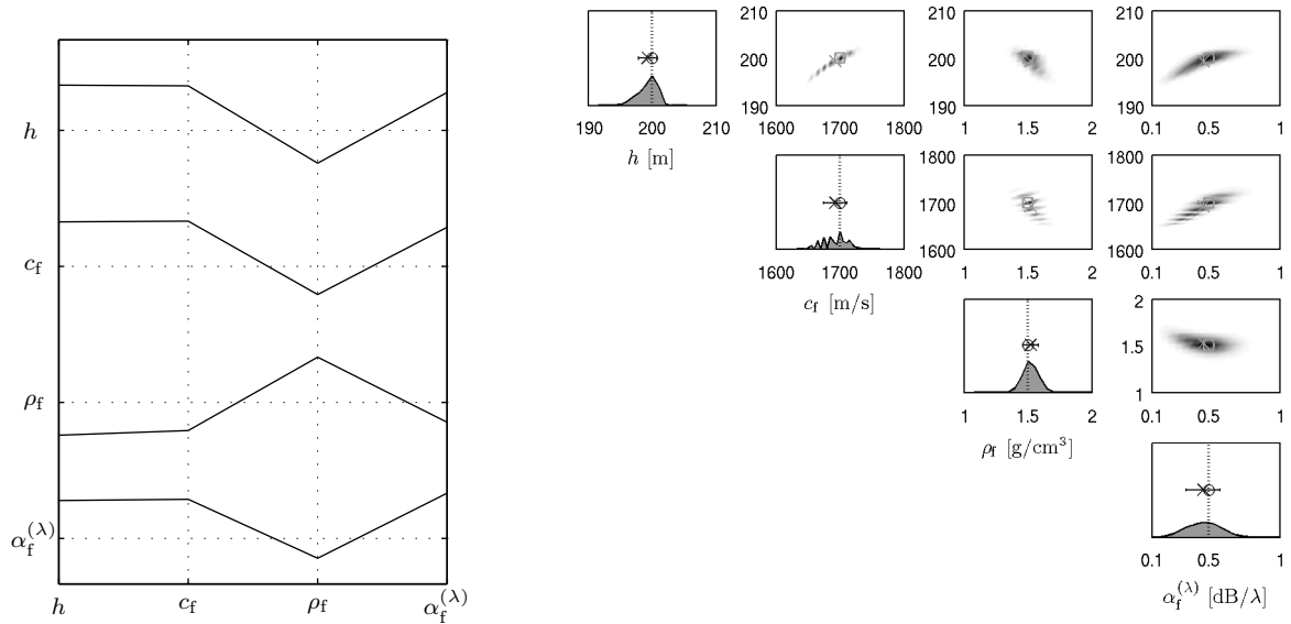
FIG. B.7 – Corrélations entre paramètres (à gauche) et densités marginales a posteriori 1D (à droite en diagonale) et 2D (à droite hors diagonale) pour une antenne verticale située à une distance de 5 km pour une fréquence de 25 Hz.
