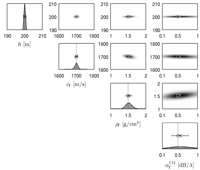
FIG. B.9 – Corrélations entre paramètres (à gauche) et densités marginales a posteriori 1D (à droite en diagonale) et 2D (à droite hors diagonale) pour une antenne verticale située à une distance de 0.5 km pour une fréquence de 50 Hz.
