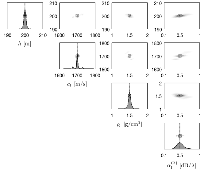
FIG. B.12 – Corrélations entre paramètres (à gauche) et densités marginales a posteriori 1D (à droite en diagonale) et 2D (à droite hors diagonale) pour une antenne verticale située à une distance de 10 km pour une fréquence de 50 Hz.
