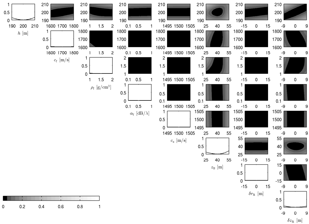
FIG. A.5 – Coupes 1D (en diagonale) et 2D (hors diagonale) du corrélateur de Bartlett pour une antenne verticale située à une distance de 500 m et pour une fréquence de 25 Hz.
