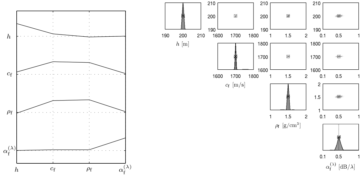
FIG. B.16 – Corrélations entre paramètres (à gauche) et densités marginales a posteriori 1D (à droite en diagonale) et 2D (à droite hors diagonale) pour une antenne verticale située à une distance de 10 km pour une fréquence de 100 Hz.
