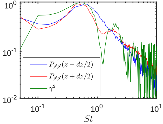
FIGURE 5.15 – Spectres et cohérence mesurés en deux points séparés axialement de 0.42D autour de z = 3D à y = 0.4D dans un jet à M_j = 0.9 .
