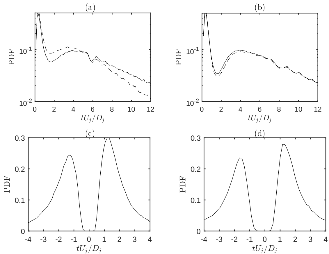
FIGURE 5.32 – (a) et (b) : Densité de probabilité du délai entre deux événements de pression positifs (—) and négatifs (---). (c) et (d) : Densité de probabilité entre un pic positif et le pic négatif le plus proche. (a)-(c), M_j = 0.9 ; (b)-(d), M_j = 1.32 .
