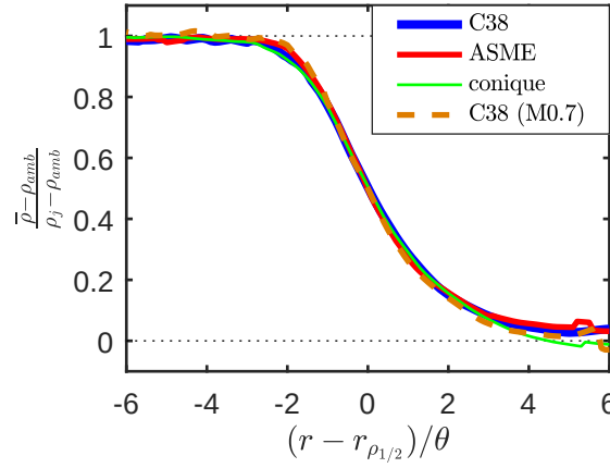
FIGURE 4.12 – Profils de masse volumique normalisés par l'épaisseur de quantité de mouvement moyenné pour chaque position disponible, et dans tous les cas testés.
