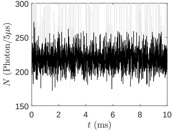
FIGURE 3.23 – Exemple d'un flux de photons échantillonné à 200 kHz. —, signal brut ; —, signal nettoyé par la méthode 2.
