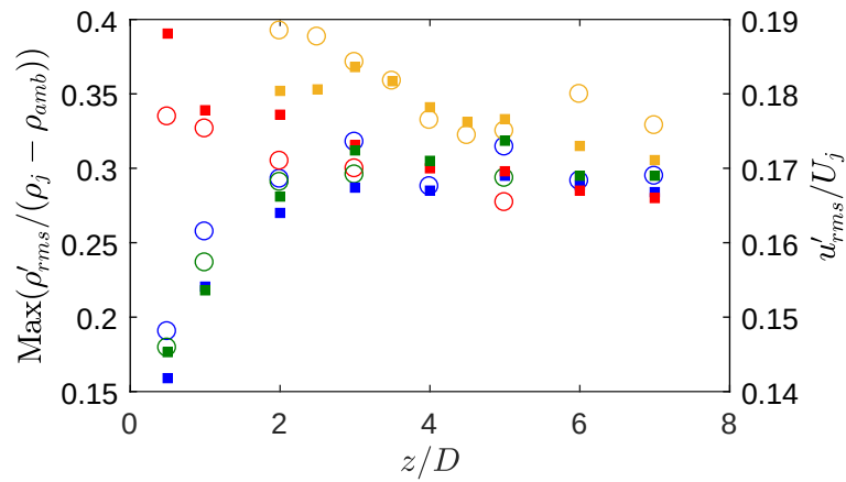
FIGURE 4.20 – Maxima des fluctuations de masse volumique (○) et de vitesse axiale (□) en fonction de la position axiale. M_j = 0.9 : ●, tuyère C38; ●, tuyère ASME; ●, tuyère conique. M_j = 0.7 : ●, tuyère C38.
