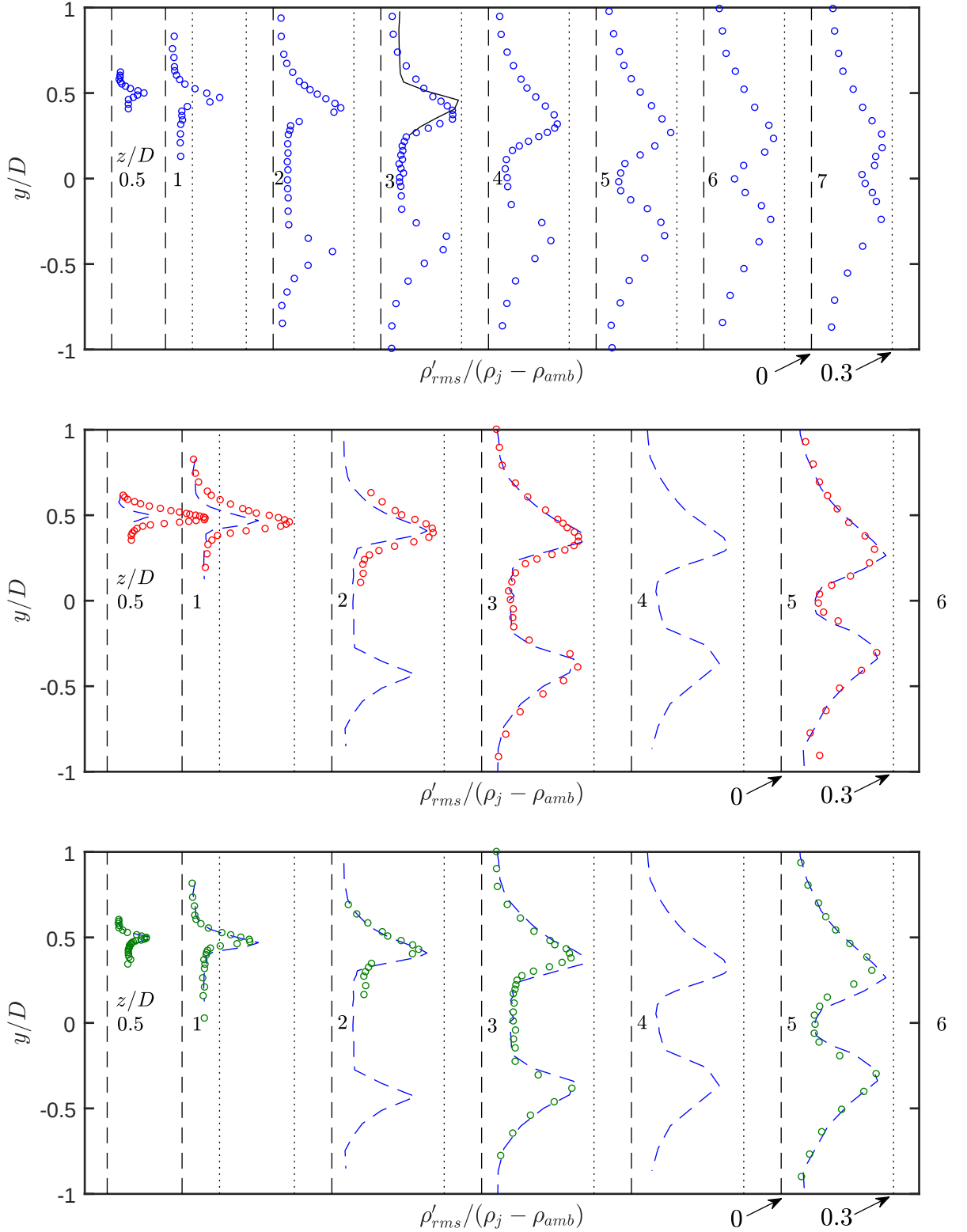
FIGURE 4.17 – Profils normalisés des fluctuations de masse volumique. M_j = 0.9 , T_0 \simeq 30^\circ\text{C} , T_{amb} \simeq 20^\circ\text{C} . \circ et - - , tuyère C38; \circ , tuyère ASME, \circ , tuyère conique. —, mesures de Panda [69] dans un jet à Mach 0.9 froid.
