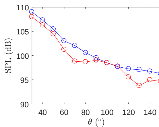
FIGURE 5.23 – Niveau acoustique produit par un jet à M_j = 0.9 mesuré sur l'antenne de directivité, sans châssis (—), et avec (—).
