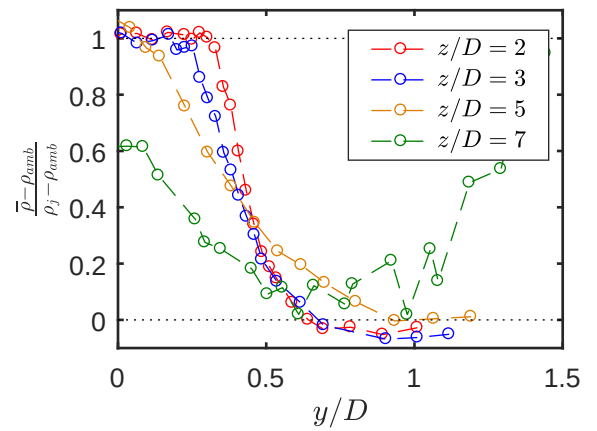
FIGURE 4.7 – Profils radiaux de masse volumique normalisés, mesurés dans un jet à Mach 0.7 issu de la tuyère C38. En moyenne \rho_{amb} = 1.18 \text{ kg/m}^3 et \rho_j = 1.25 \text{ kg/m}^3
