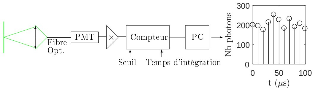
FIGURE 3.5 – Schéma d'une chaîne d'acquisition classique
