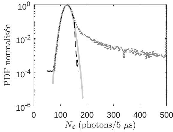
FIGURE 3.22 – Densité de probabilité : \cdots , flux de photons \Phi_d brute ; --- , flux de photons corrigé ; — distribution gaussienne.
