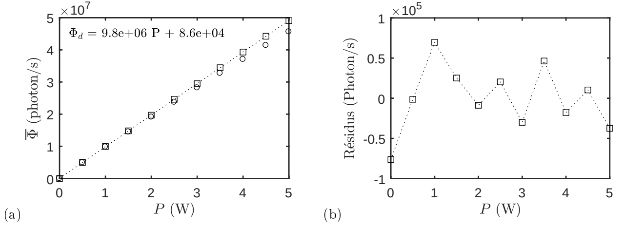
FIGURE 3.18 – (a) : flux de photons compté \Phi_c (o) en fonction de la puissance incidente, et flux collecté \Phi_d ( \cdot □ \cdot ) corrigé avec \tau = 1.6 ns. Les pointillés correspondent à la régression linéaire pour \Phi_d . (b) : différence entre \Phi_d et sa régression linéaire.
