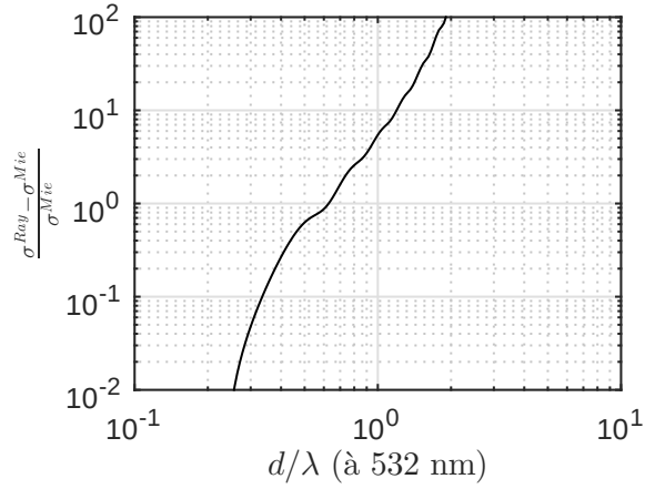
FIGURE 2.4 – Erreur relative entre le modèle de diffusion de Rayleigh et de Mie en fonction du diamètre normalisé pour des particules sphériques et homogènes.
