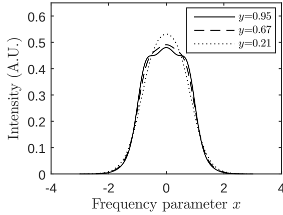
FIGURE 2.6 – Intensité arbitraire en fonction de la fréquence adimensionnelle de la diffusion Rayleigh-Brillouin spontanée dans de l’air, calculée à pression atmosphérique à l’aide du modèle de Witschas. — — — T=223\text{K} , — — — T=293\text{K} , \dots T=773\text{K}
