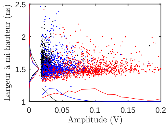
FIGURE 3.10 – Répartition des largeurs de pulse en fonction de l'amplitude pour \dots , V_{cont} = 0.7 V ; \dots , V_{cont} = 0.8 V ; \dots , V_{cont} = 0.9 V. Les lignes représentent les densités de probabilités dans leurs axes respectifs.
