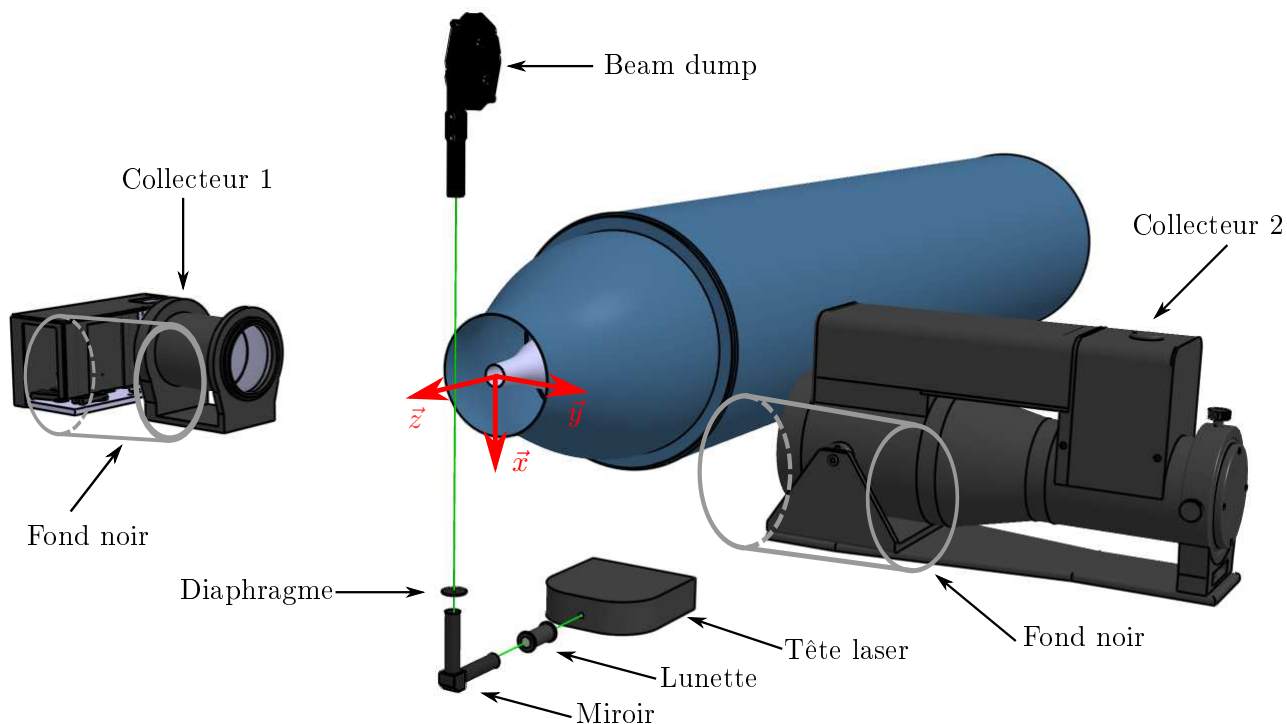
FIGURE 3.1 – Représentation des différents éléments du dispositif de mesure. Les échelles sont respectées.
